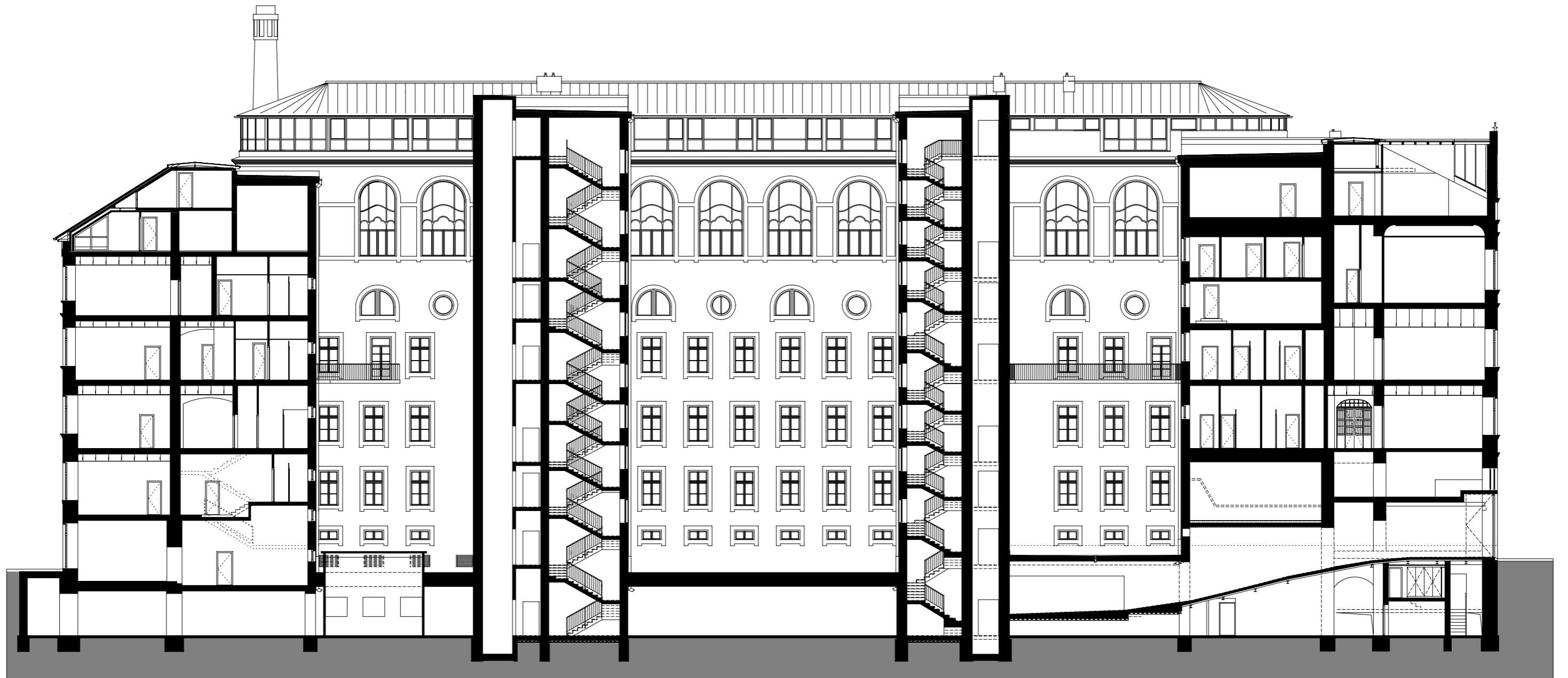
HOSSZMETSZET A LÉGUDVAROKON ÁT
