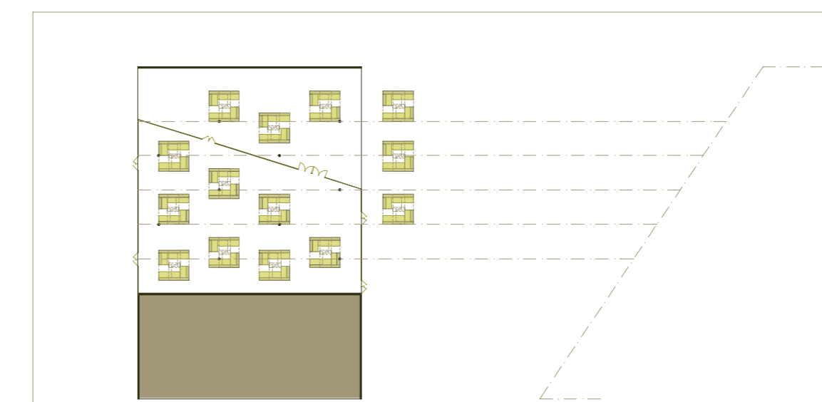
virágpiac berendezési változatai - szigetyszerű elrendezés A rajz a burkolt felület 3,00 x 1,00 (+1,00) m nagysági árusítóhelyekkel történő berendezést mutatja, a virágpiac területén legalább 32, fedett-nyitott térben 12 darab stand, külterén legalább 12 darab ideiglenes stand helyezhető el.
