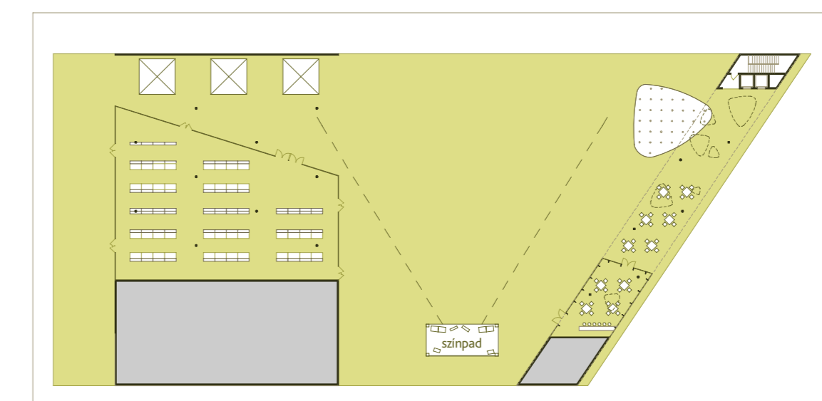
térhasználat változatai - kulturális rendezvény A rajz a burkolt felület színpaddal és ideiglenes árusítóhelyekkel történő berendezését mutatja, a területen legalább 2000 látogató elfér.
