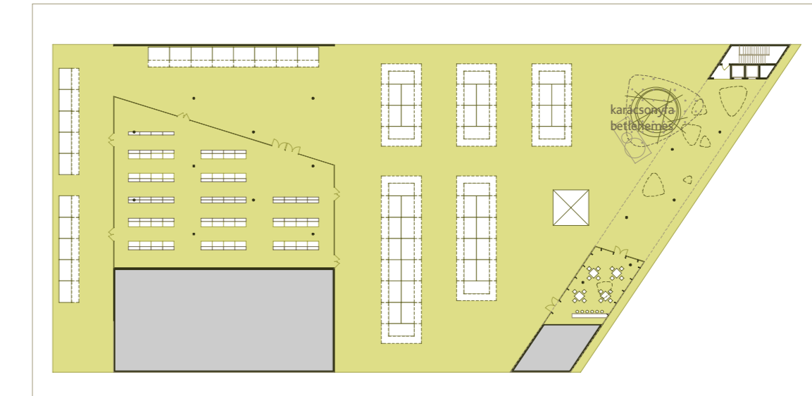
térhasználat változatai - karácsonyi vásár A rajz a burkolt felület 3,00 x 1,00 (+1,00) m nagysági ideiglenes árusítóhelyekkel történő berendezését mutatja, a területen legalább 60 pavilon helyezhető el.
