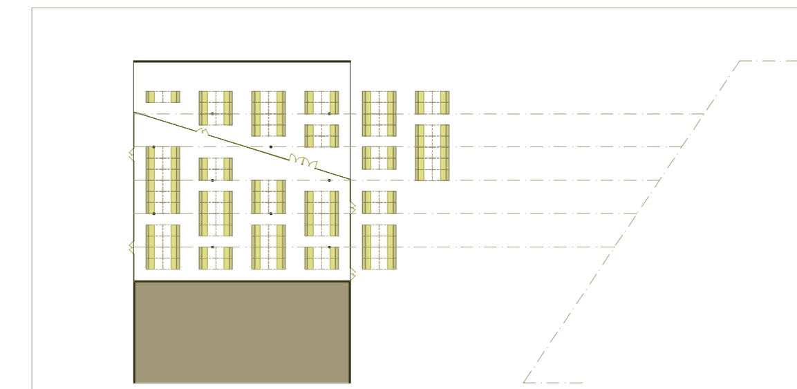
virágpiac berendezési változatai - függőleges elrendezés A rajz a 1,60 x 1,20 (+1,20) m nagysági árusítóhelyekkel történő berendezést mutatja, a virágpiac területén legalább 62, fedett-nyitott térben 24 darab stand, külterén legalább 42 darab ideiglenes stand helyezhető el.
