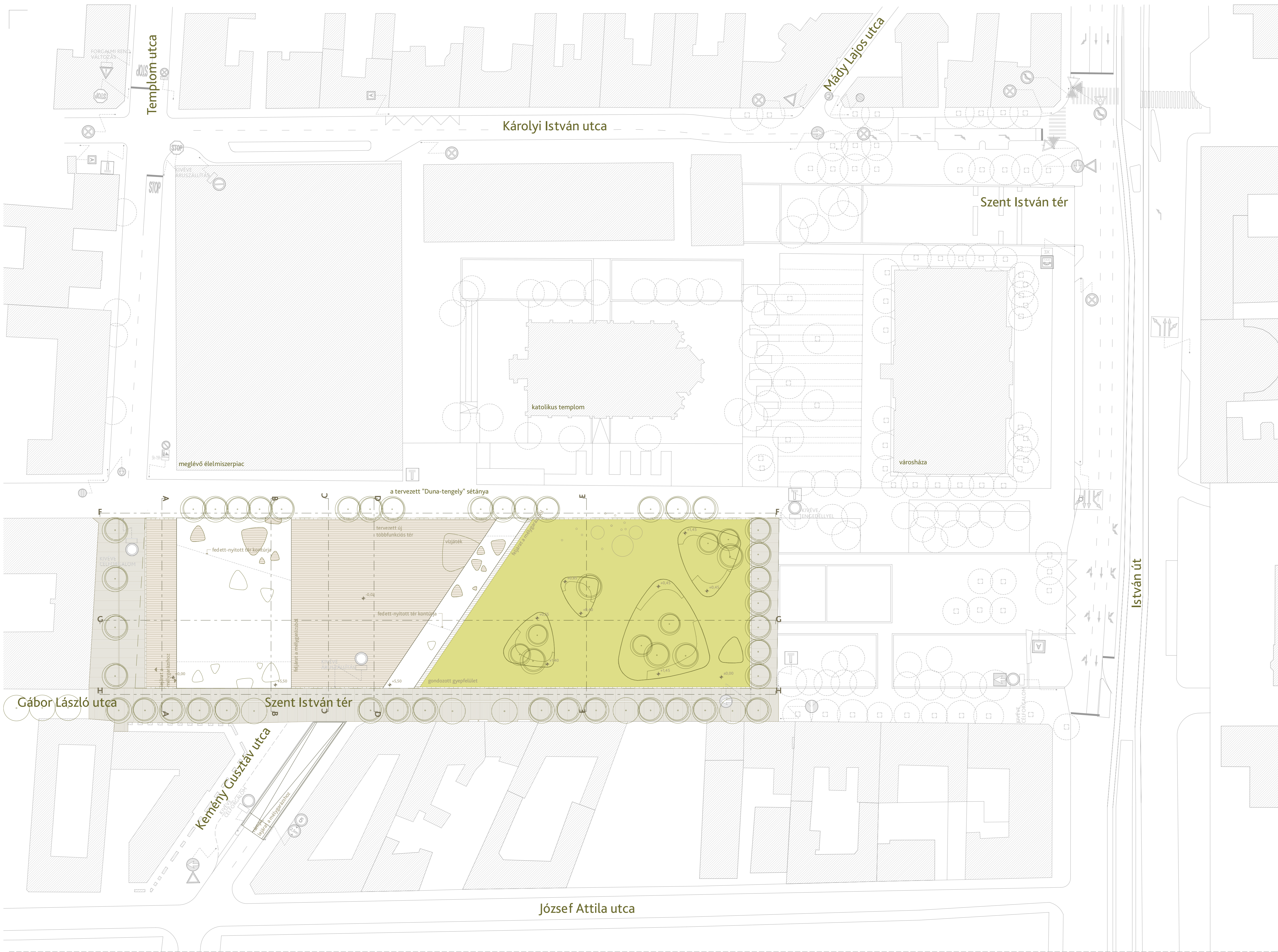
virágpiac berendezési változatai - vízszintes elrendezés A rajz a 1,20 x 1,20 (+1,00) m nagysági árusítóhelyekkel történő berendezést mutatja, a virágpiac területén legalább 56, fedett-nyitott térben 24 darab stand, külterén legalább 36 darab ideiglenes stand helyezhető el.
