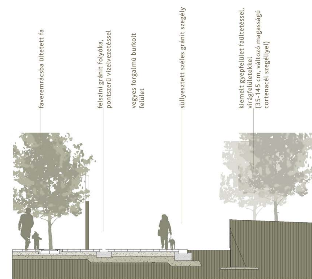
4-4 részlet
