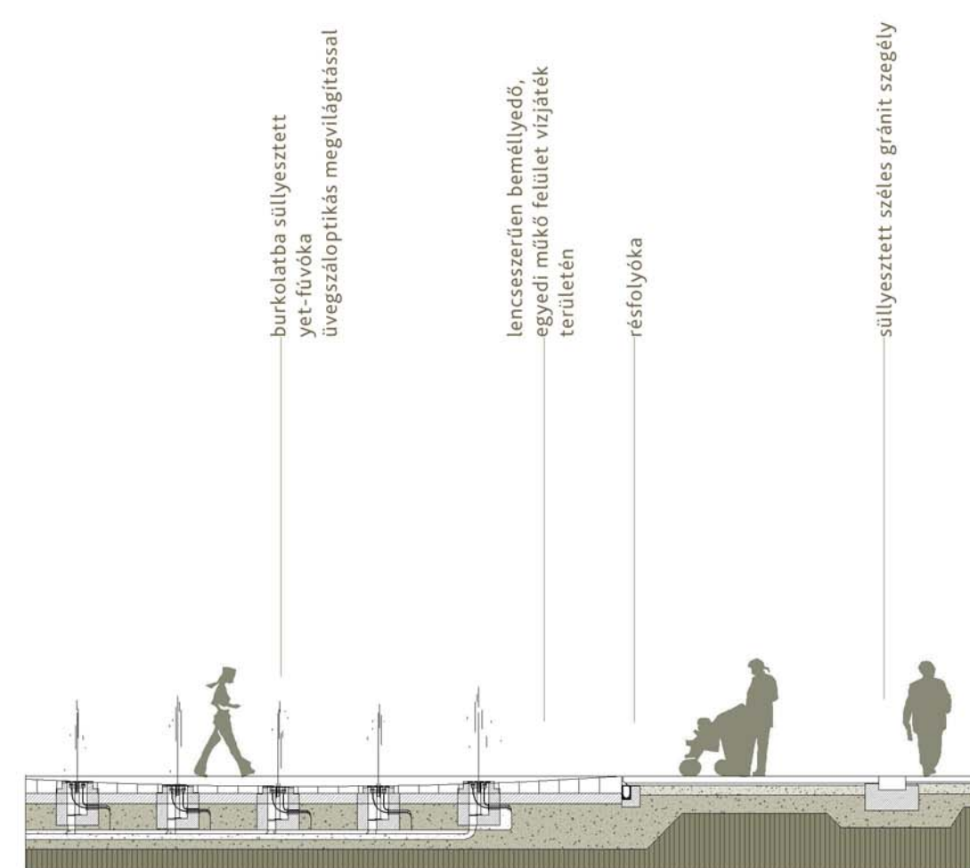
2-2 részlet
