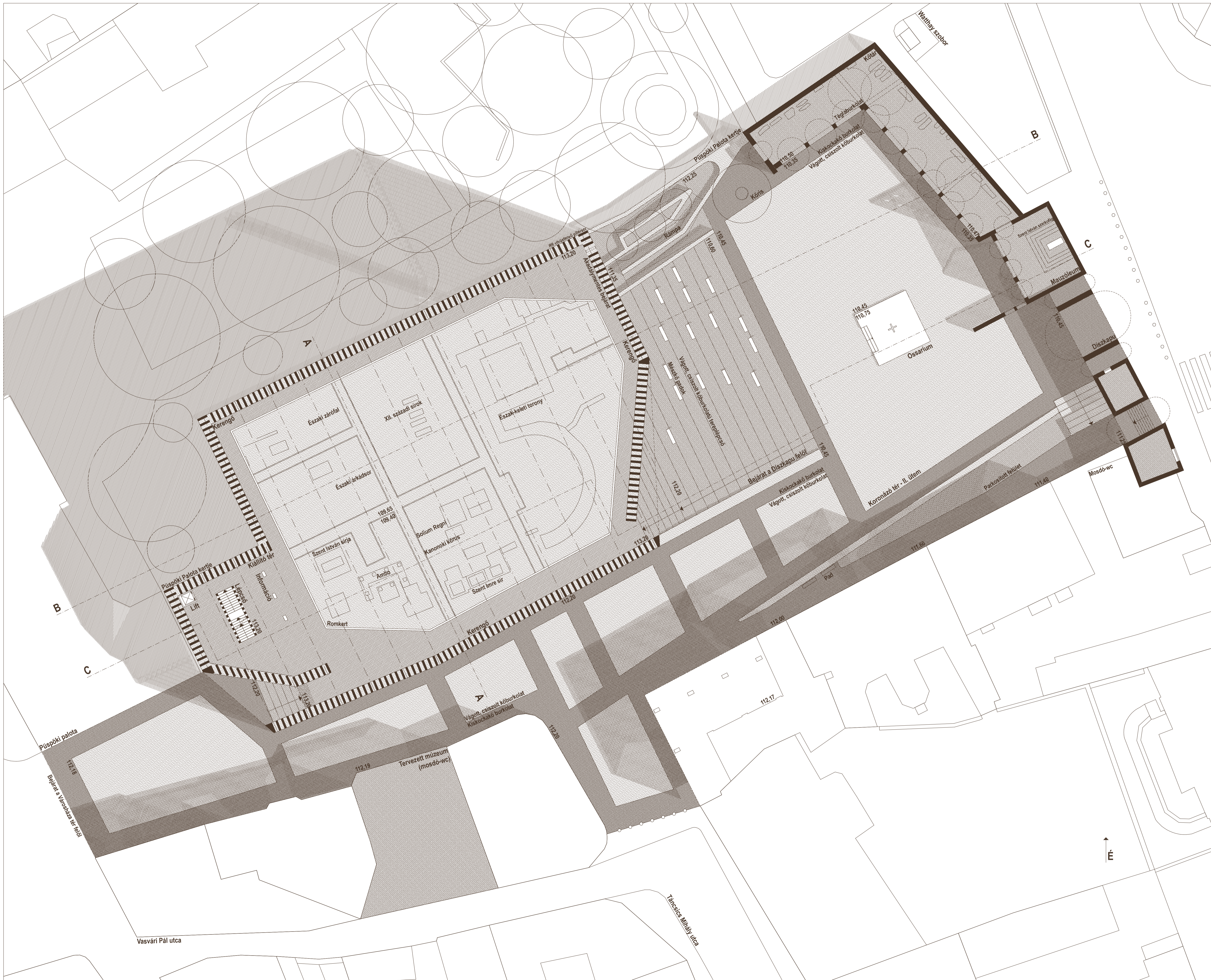
BEJÁRATI SZINT ALAPRAJZA M=1:200, ÁLTALÁNOS EMELETI ALAPRAJZ (116,70-120,20-123,70-127,20-130,70-134,20-137,70 SZINTEK) M=1:200, OSSARIUM TERVEI M=1:100 - 2/6
