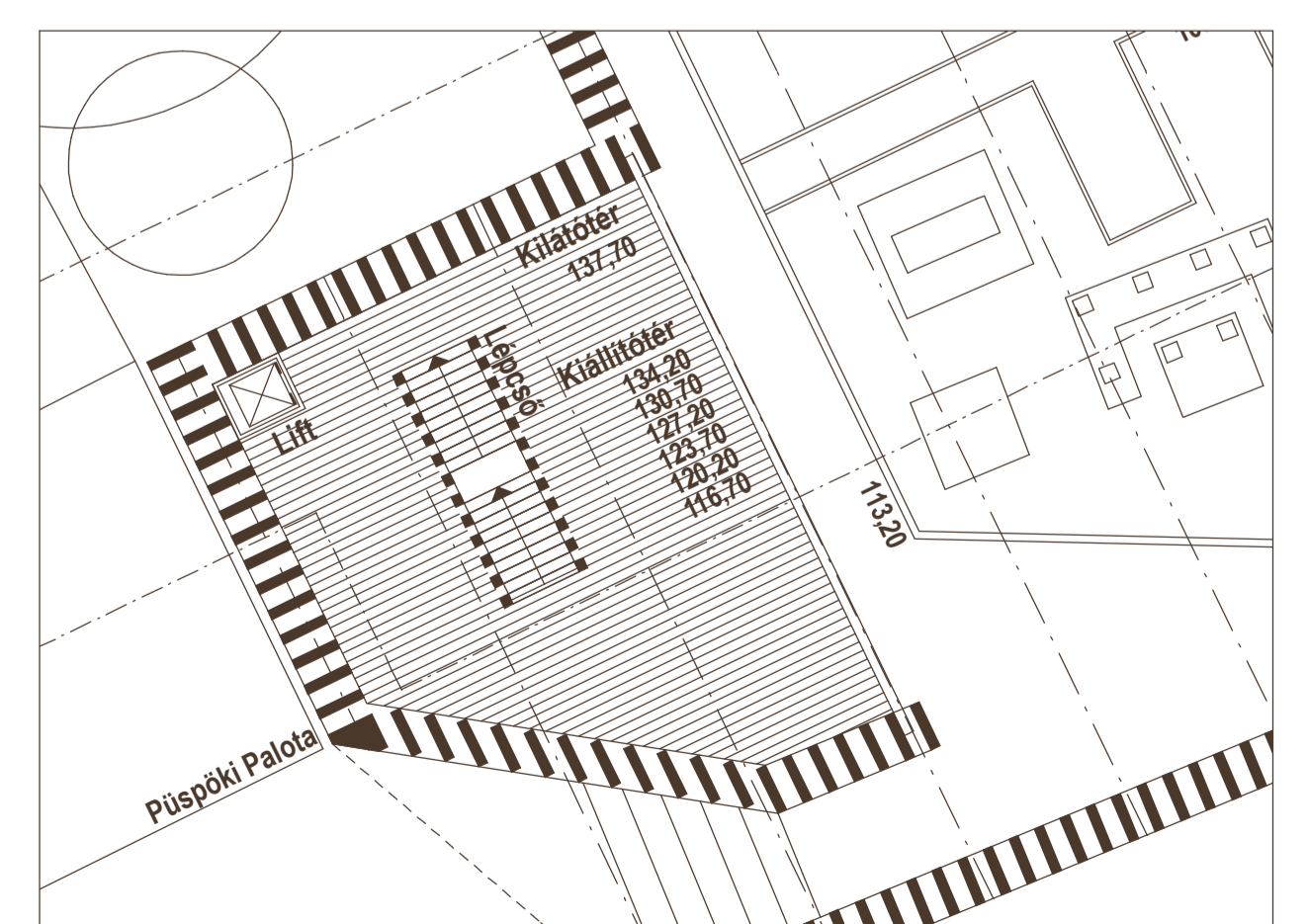
BEJÁRATI SZINT ALAPRAJZA M=1:200, ÁLTALÁNOS EMELETI ALAPRAJZ (116,70-120,20-123,70-127,20-130,70-134,20-137,70 SZINTEK) M=1:200, OSSARIUM TERVEI M=1:100 - 2/6
