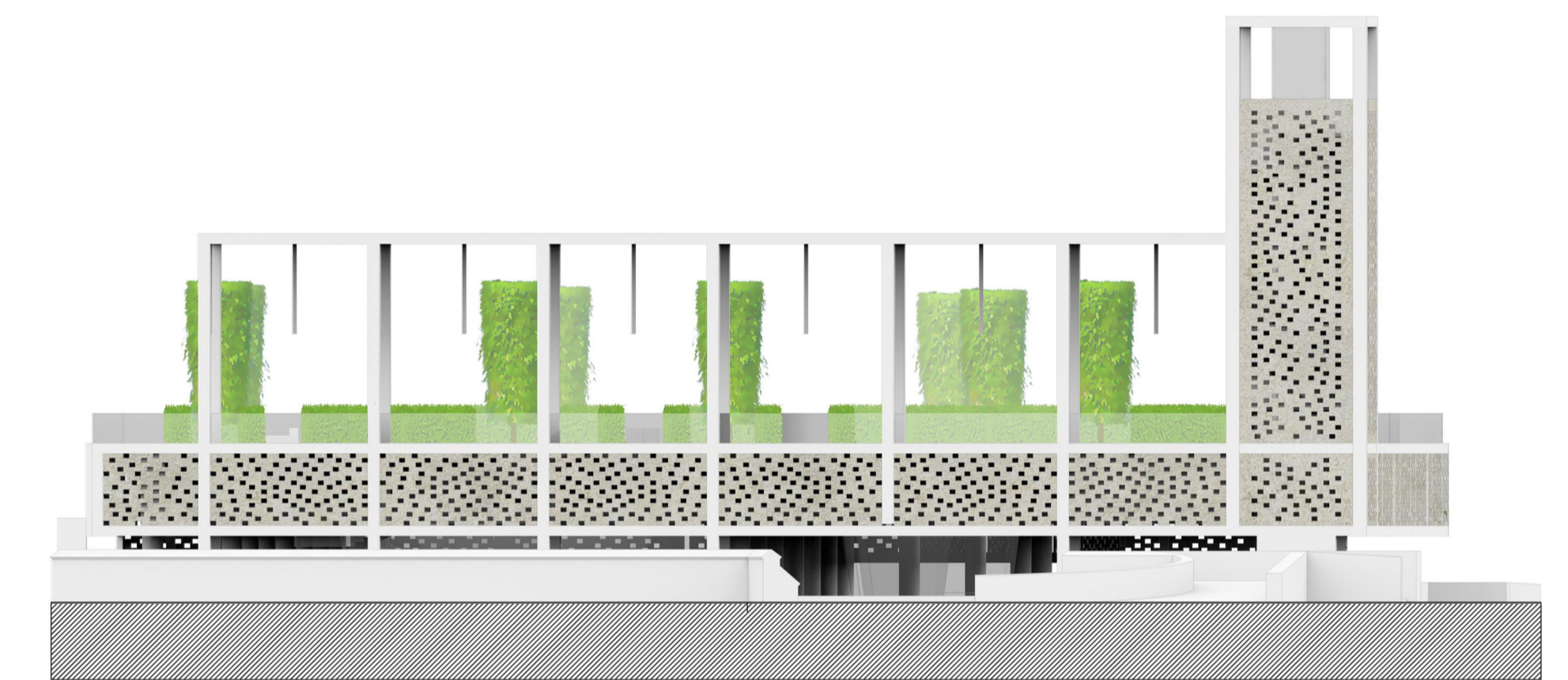
nyugati homlokzat
