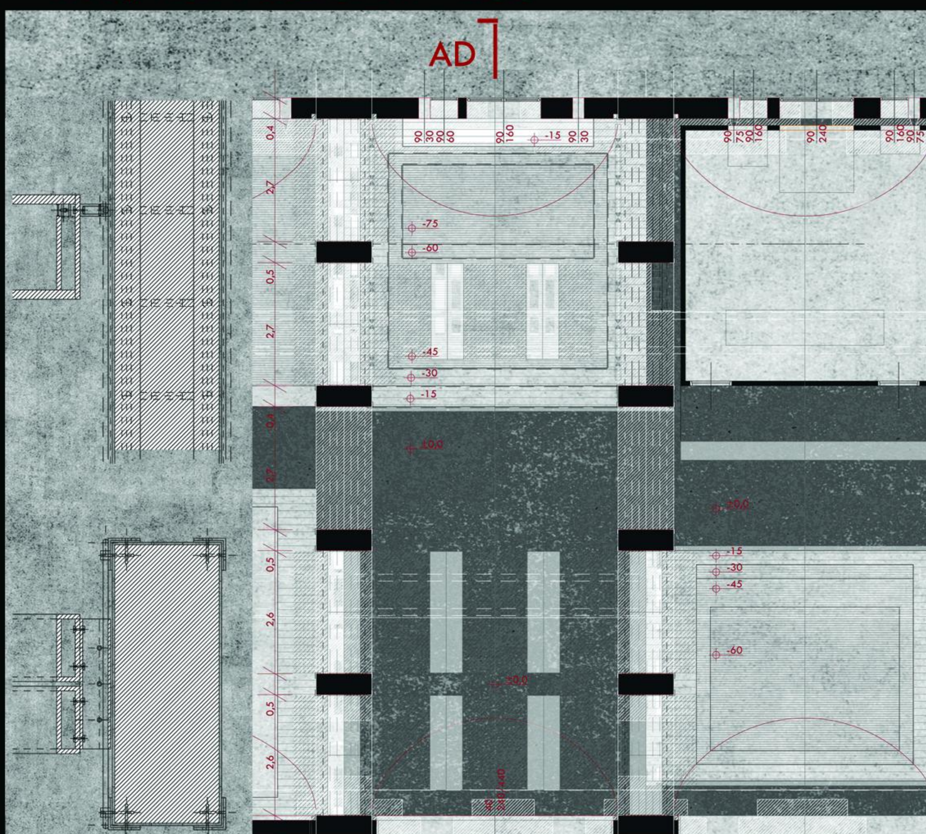
◆ variábilis könyvespolc M=1:10
