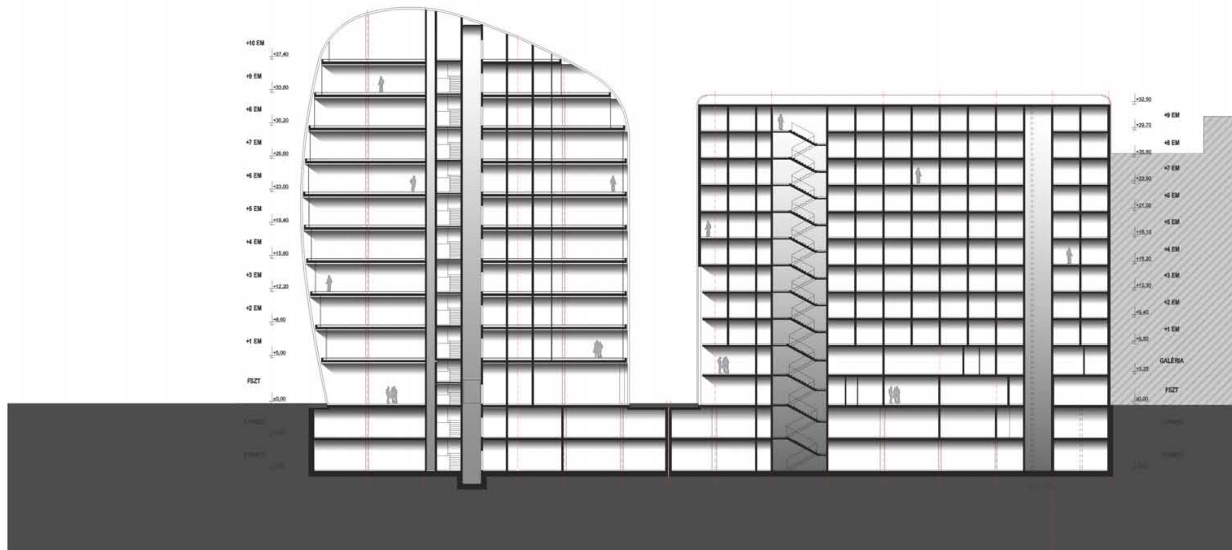
B-B METSZET
