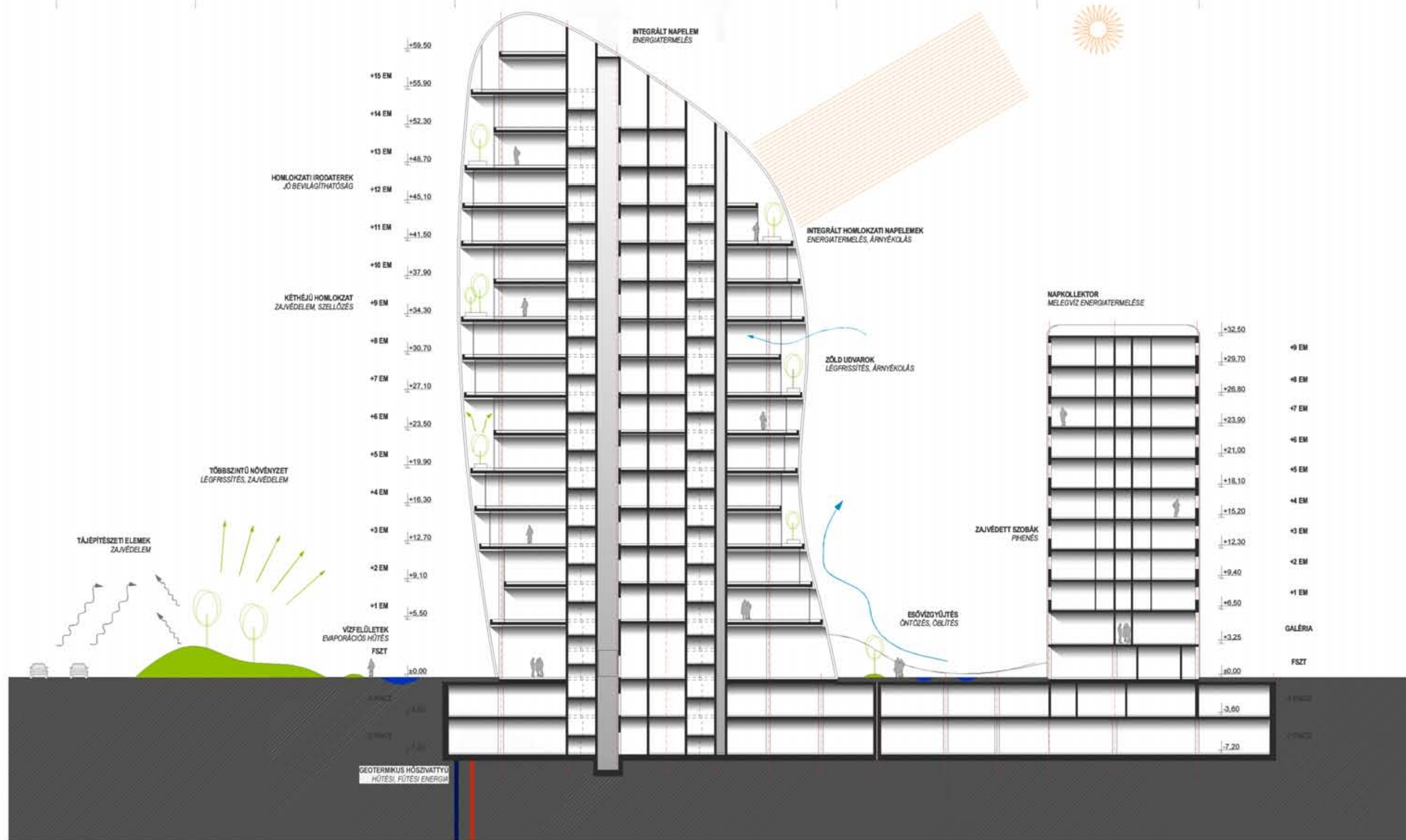
A-A METSZET
