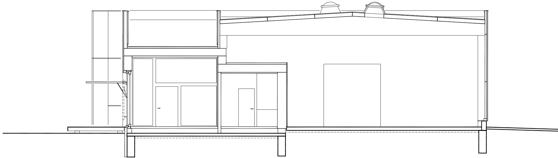
Schnitt A-A
