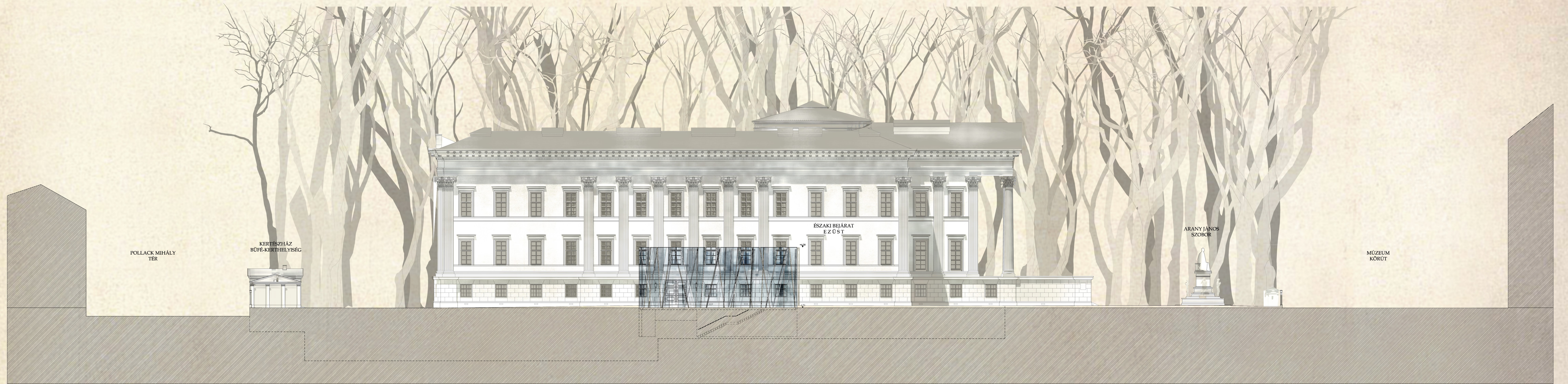
ÉSZAKI HOMLOKZAT
