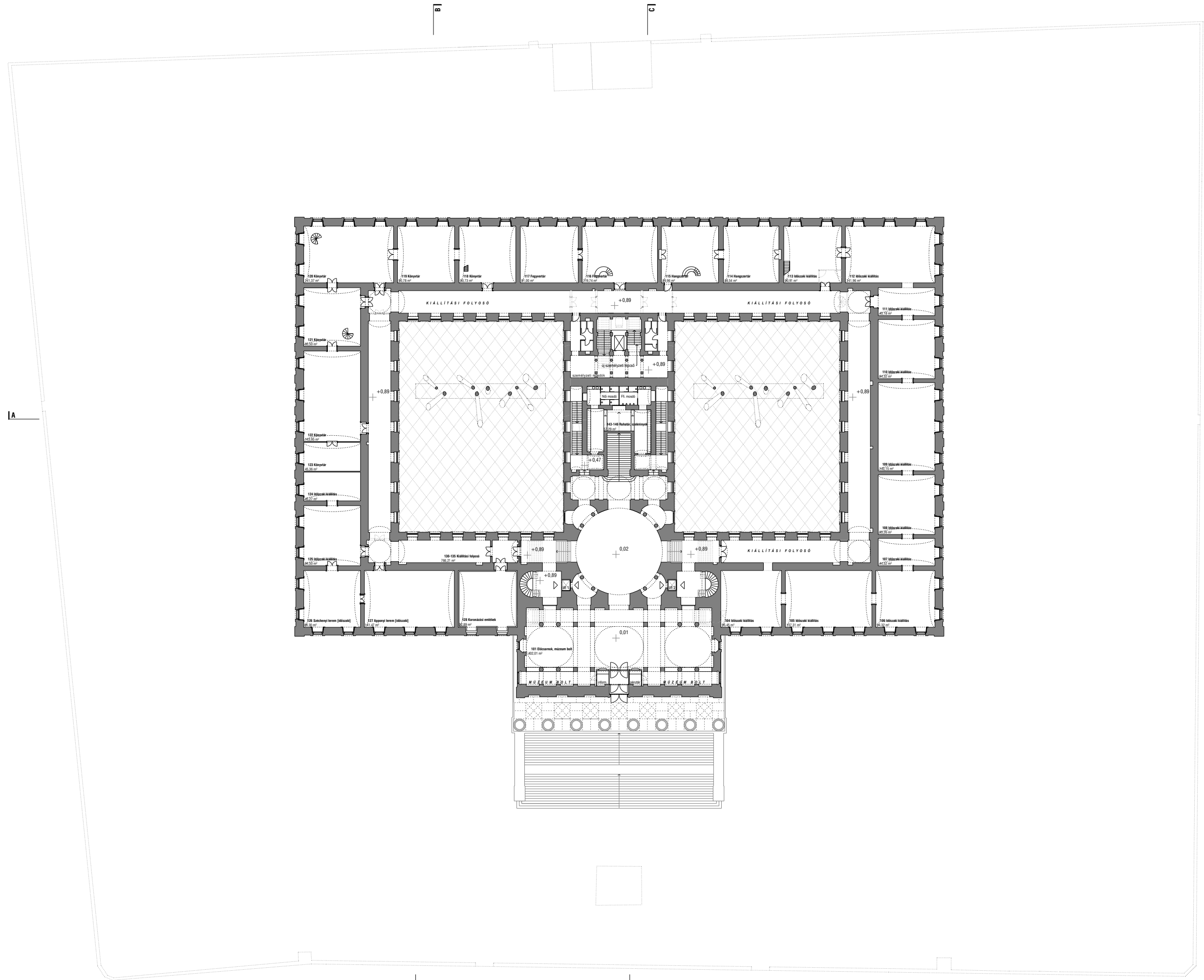
1. EMELET ALAPRAJZA_m 1:250
