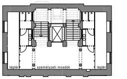
1-2. FÉLEMELET ALAPRAJZA_m 1:250
