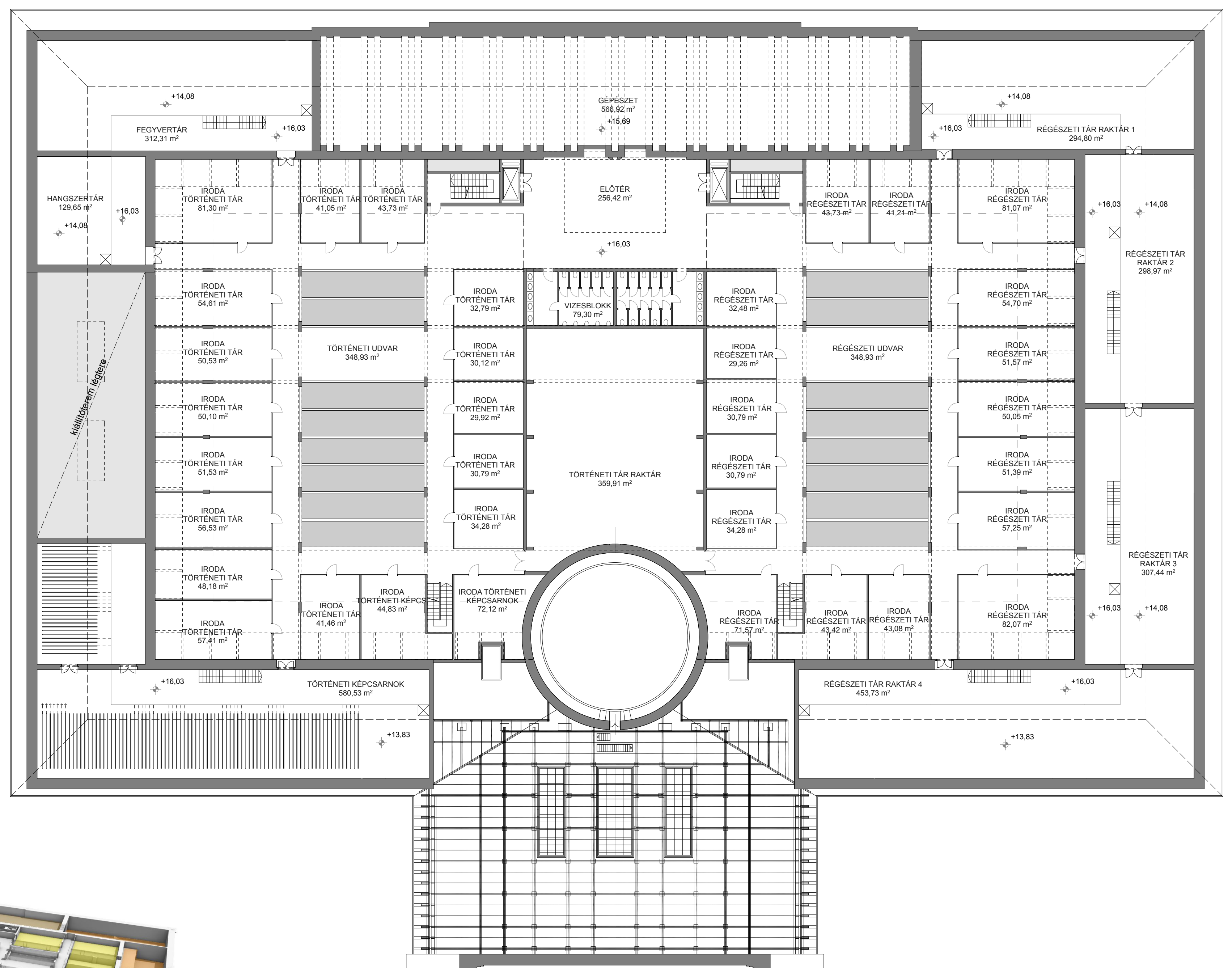
HARMADIK EMELETI ALAPRAJZ
