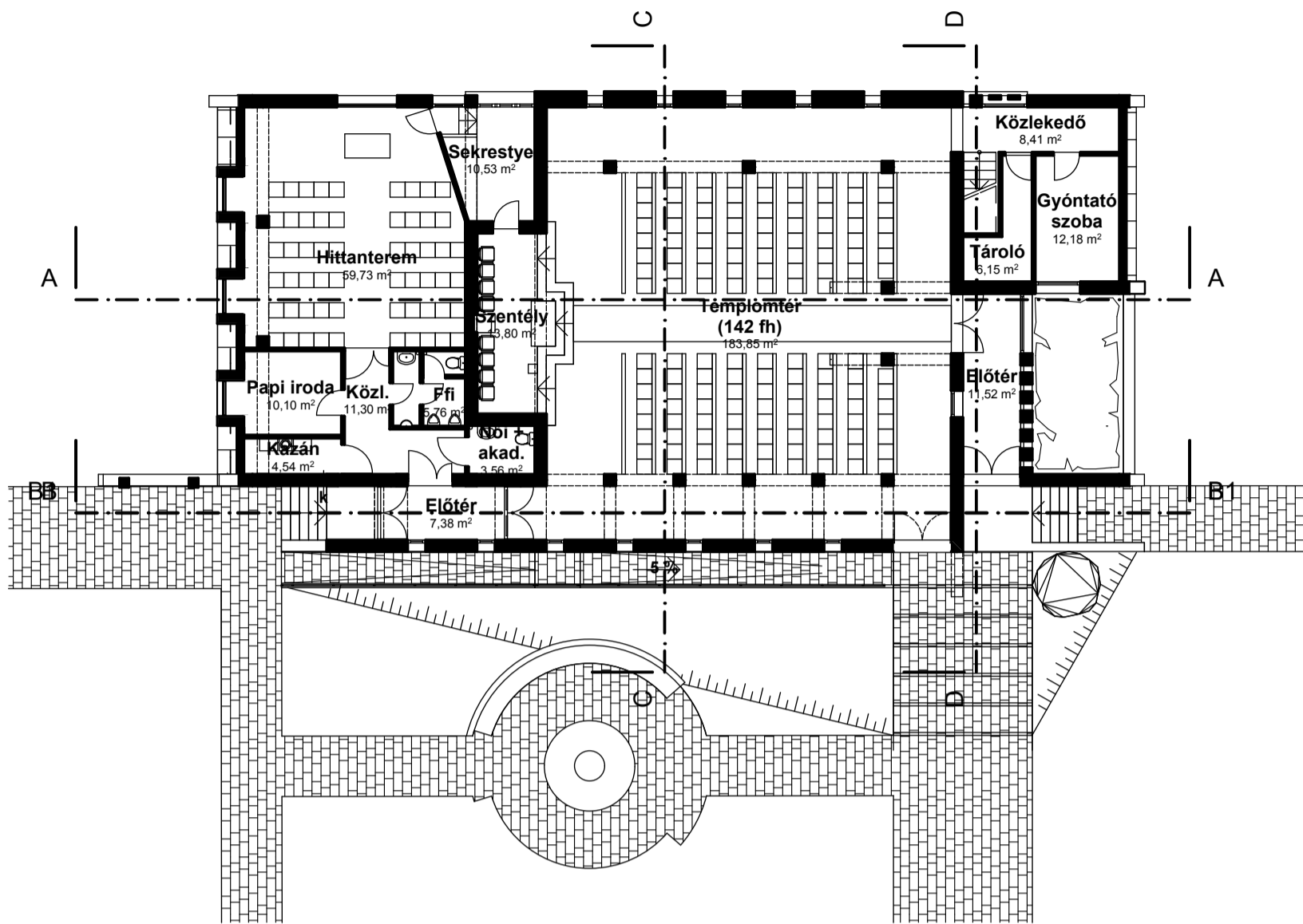
Földszinti alaprajz
