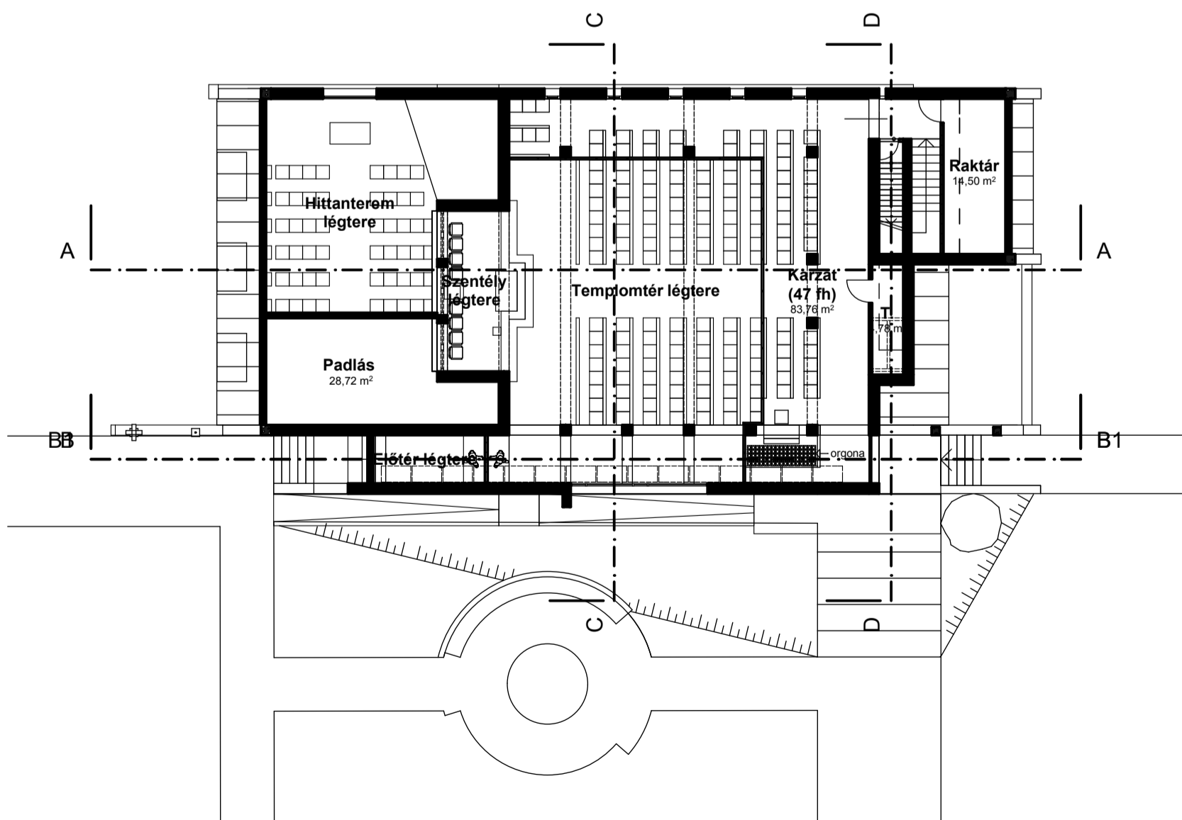
Korzatszinti alaprajz
