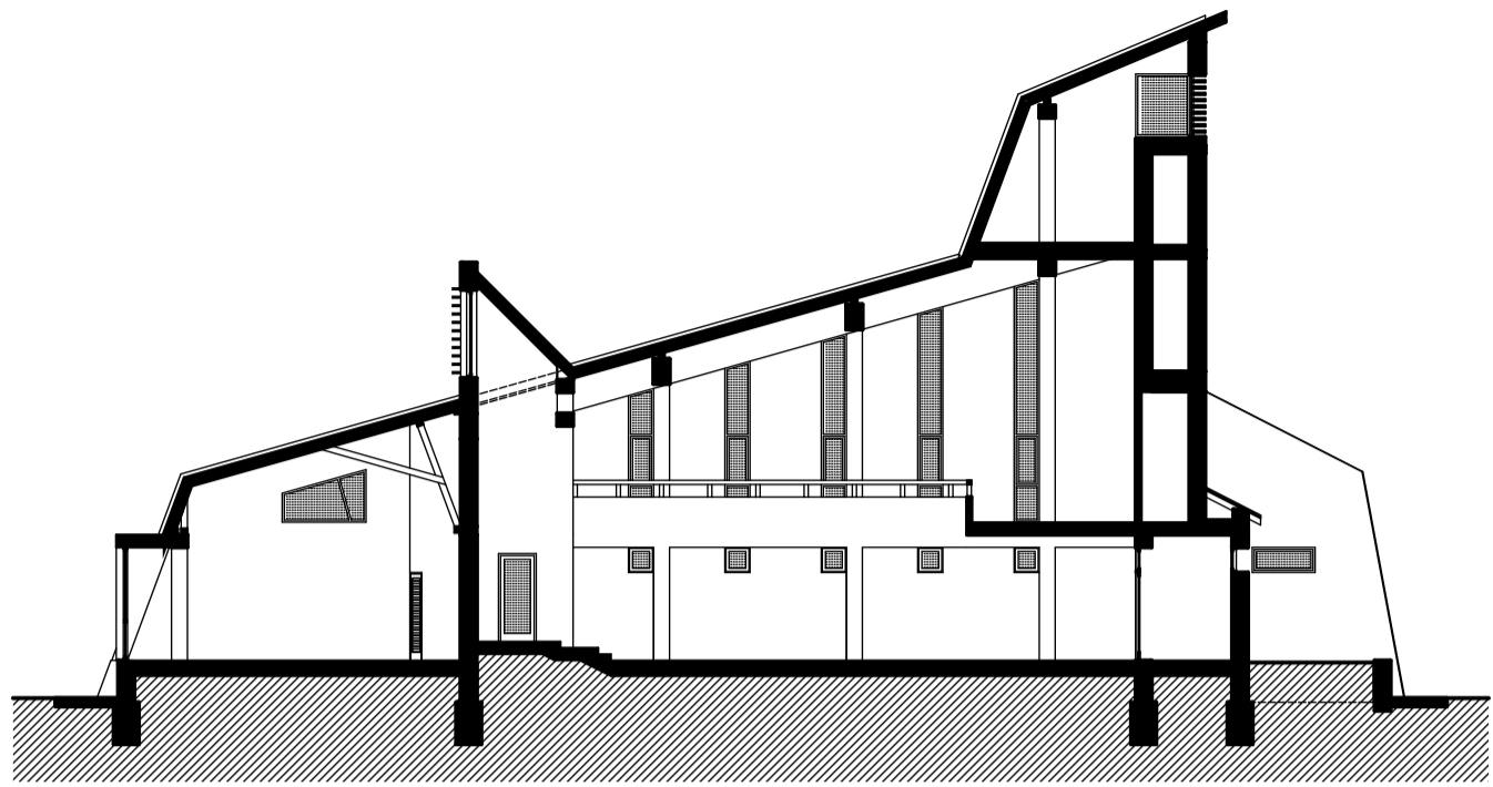
A-A metszet
