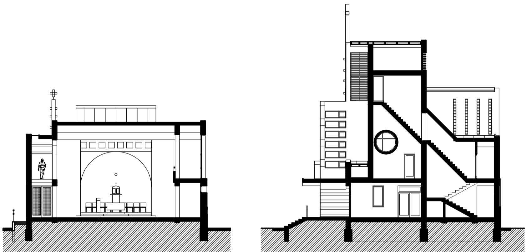
C-C metszet
