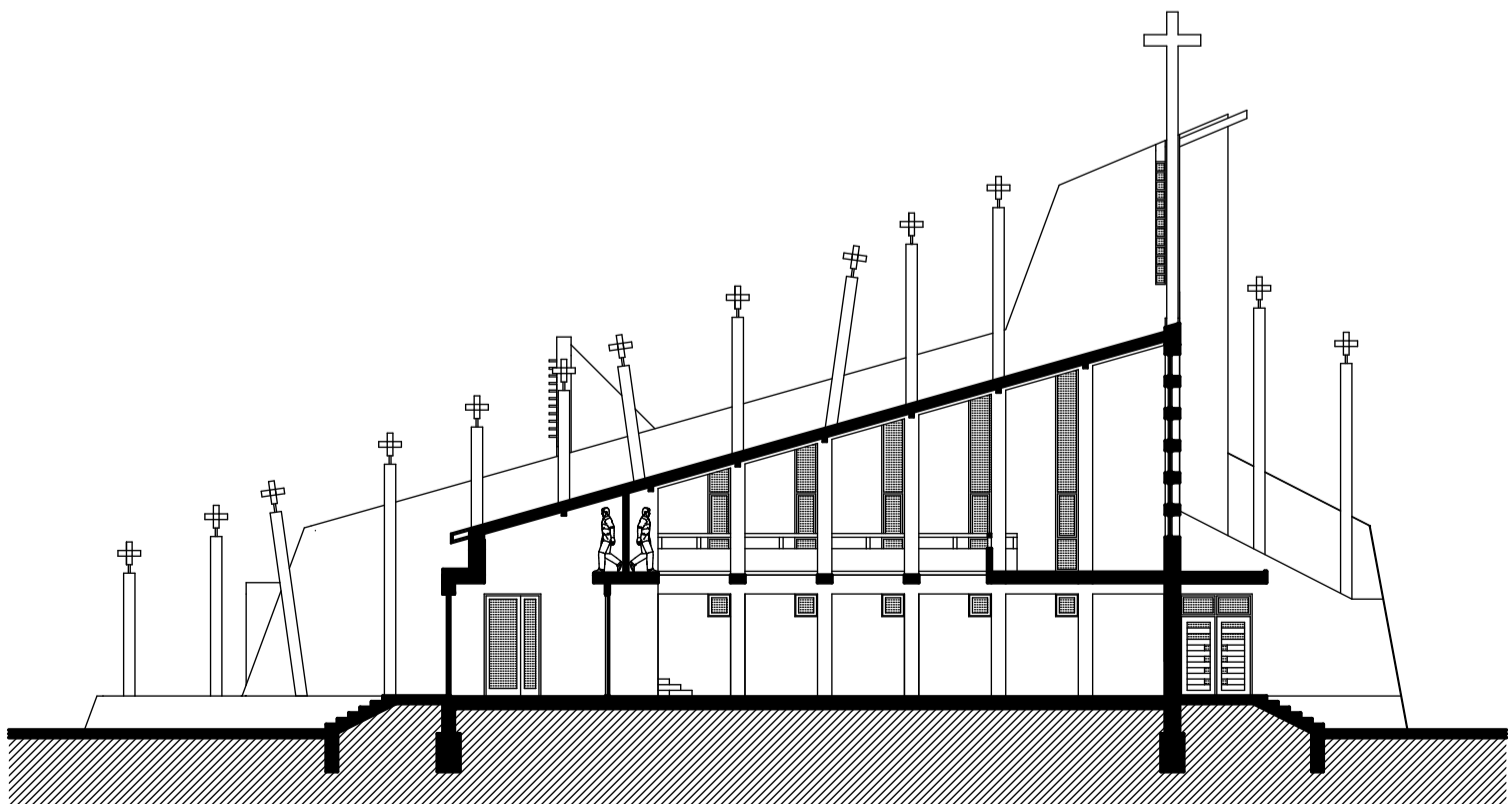
B-B metszet
