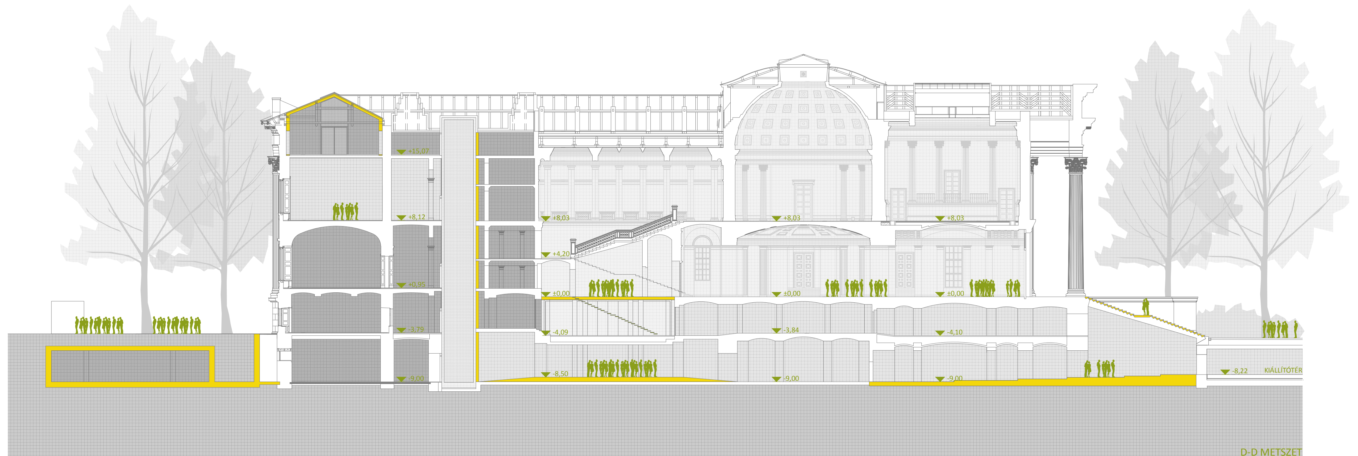
D-D METSZET
