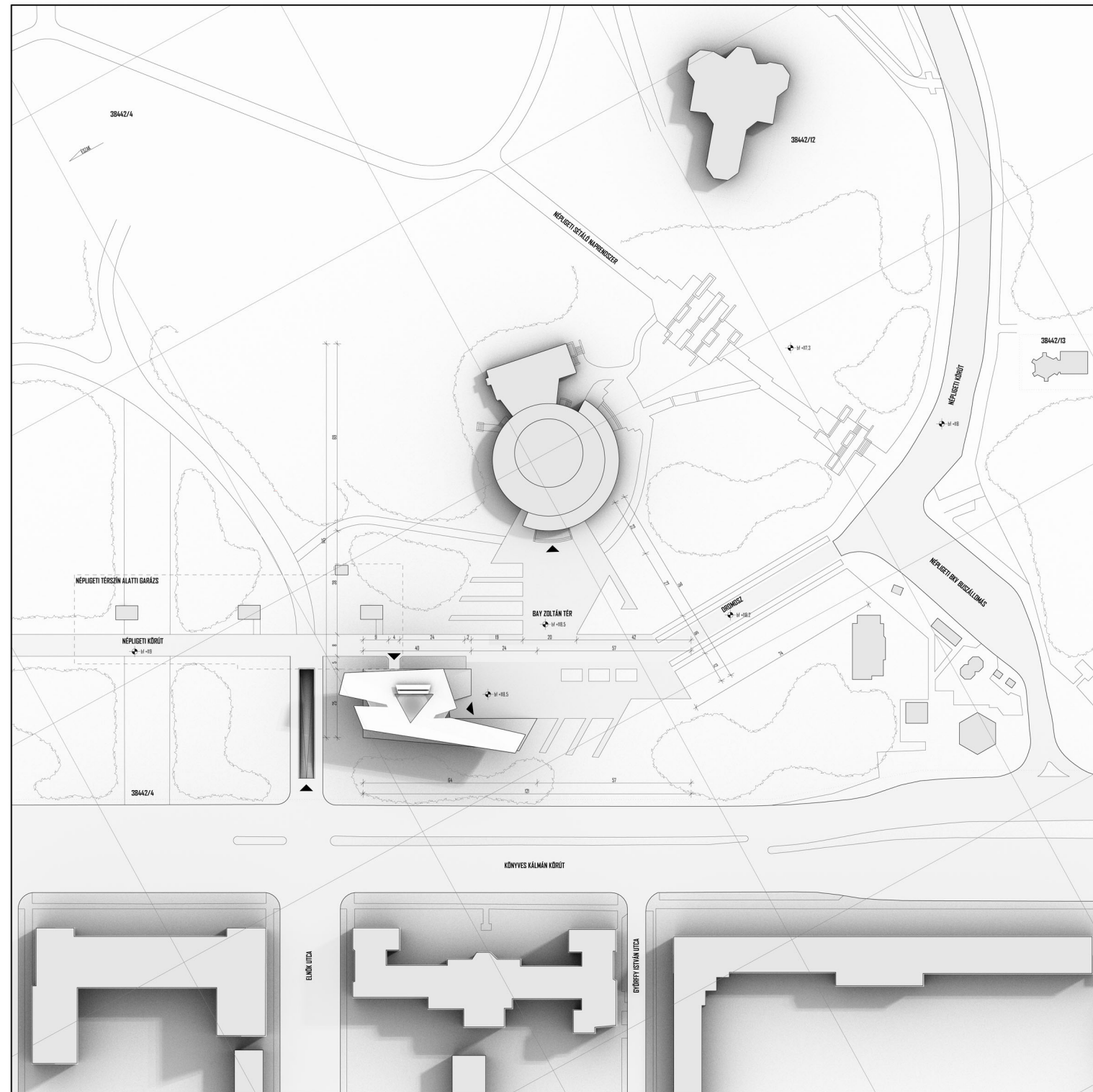
HELYSÍNRAJZ M:1/1000
