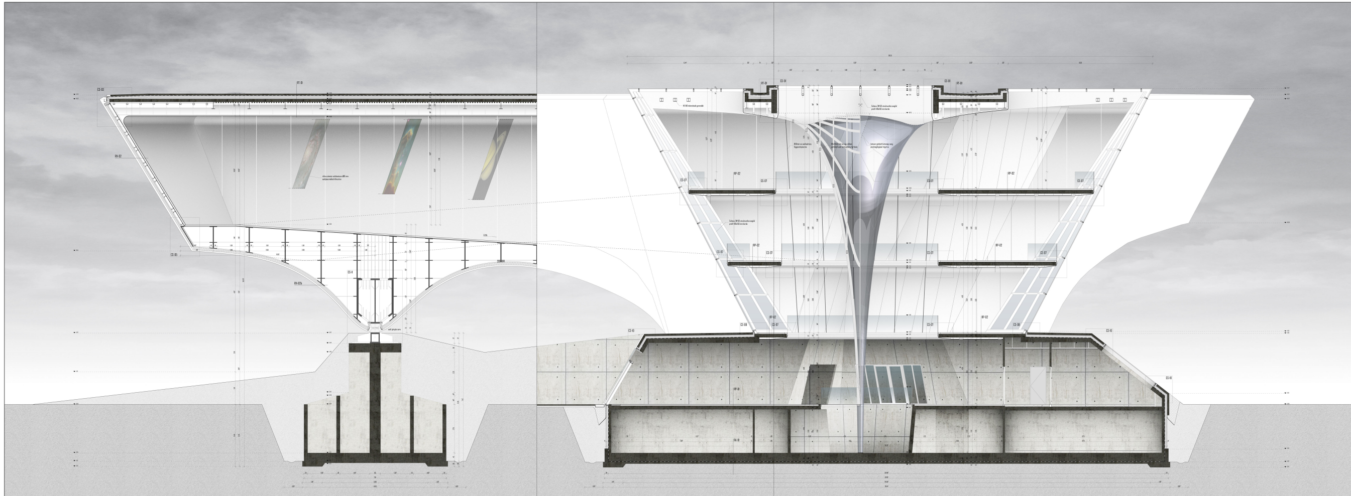
A-A METSZET M.1/50
