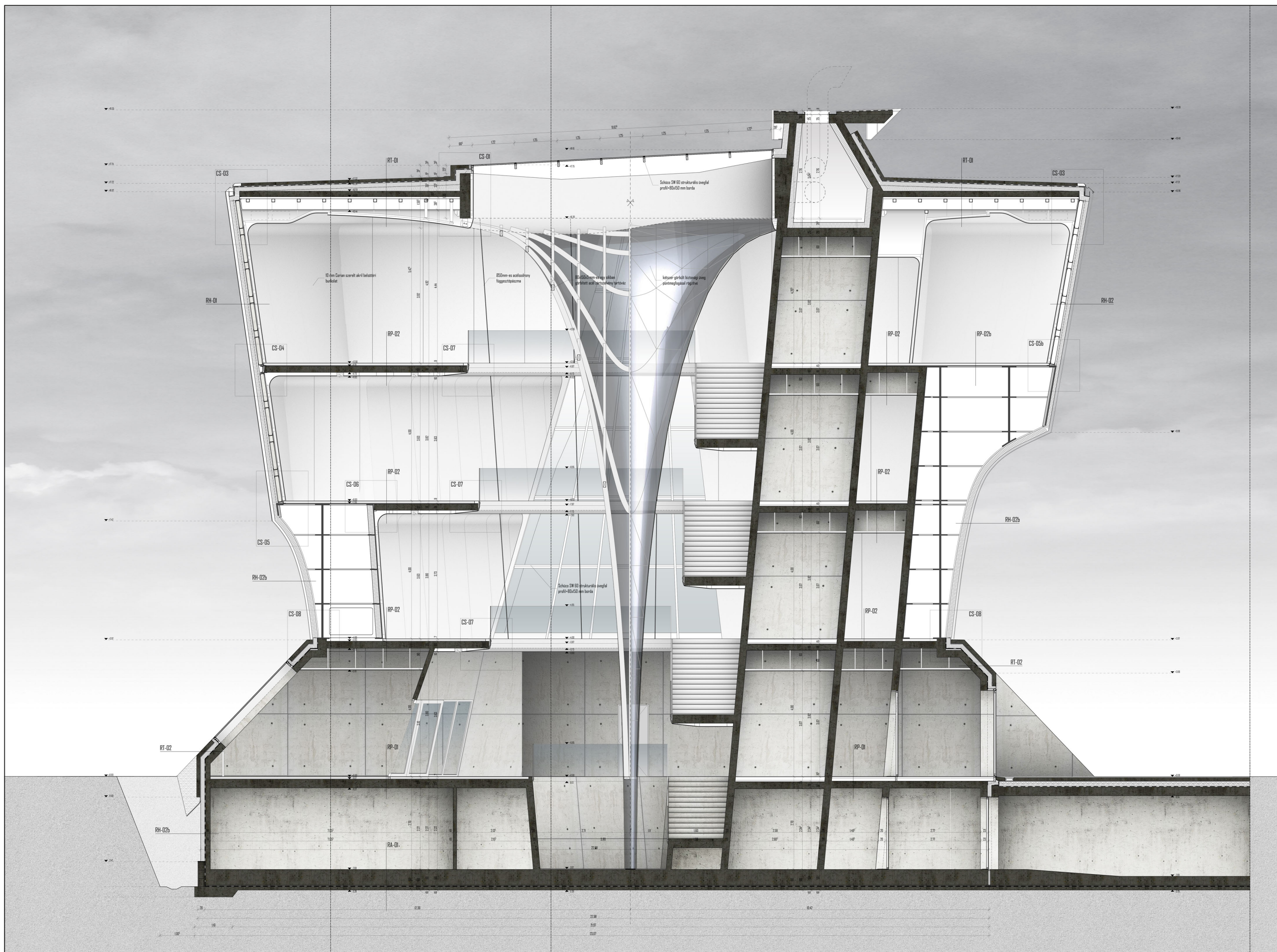
B-B METSZET M:1/50
