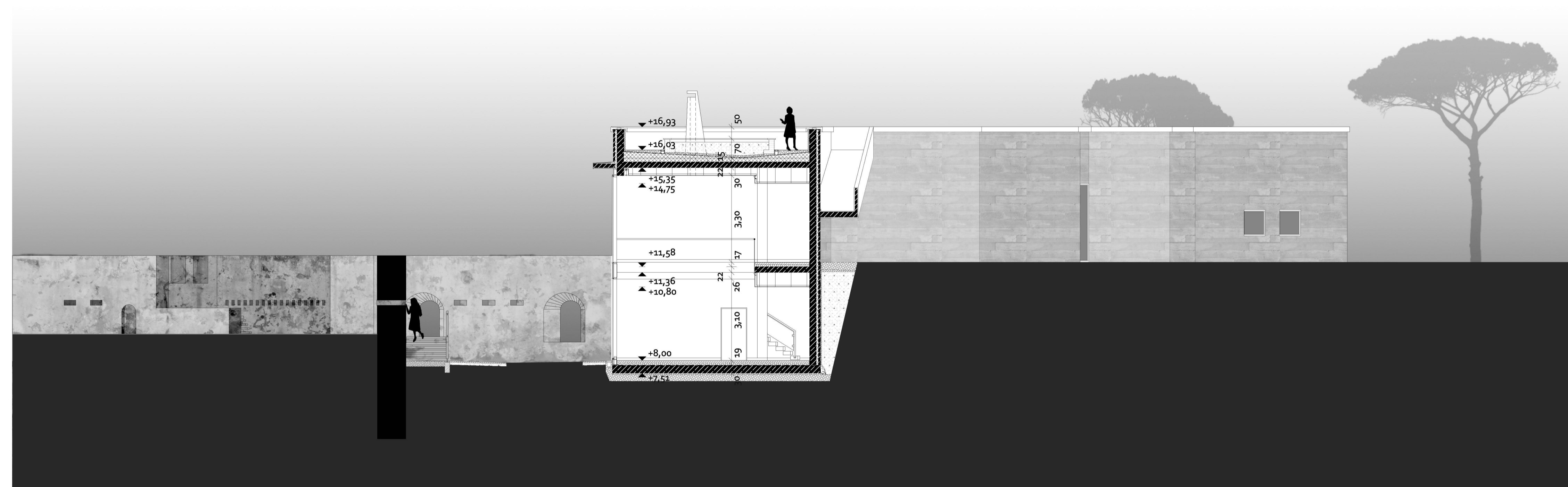
D-D METSZET
