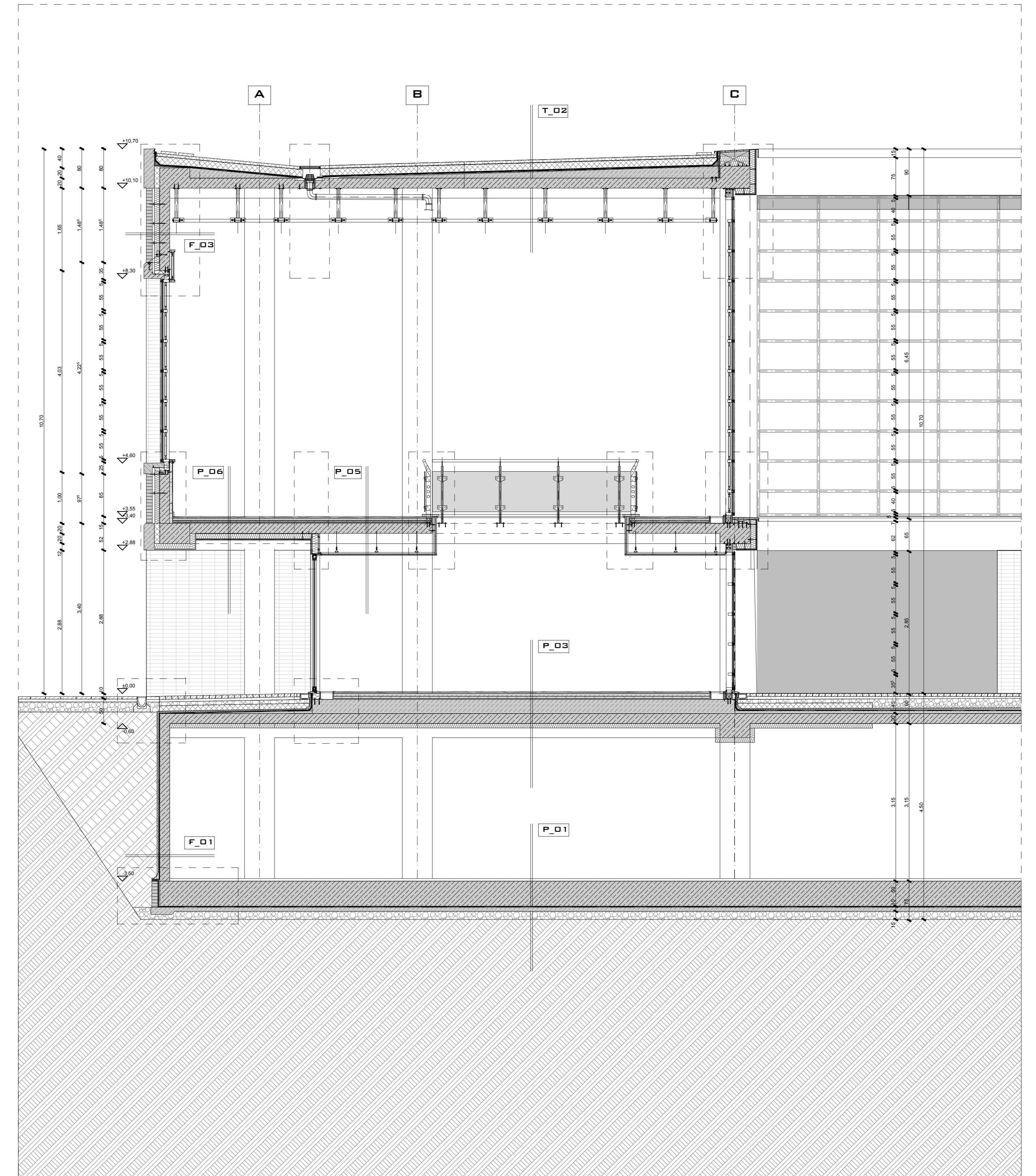
AZ ELŐCSARNOK RÉSZLETES METSZETE M=1:50
