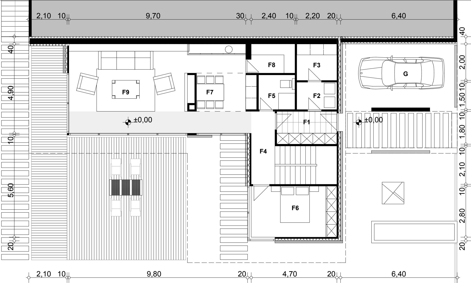
FÖLDSZINTI ALAPRAJZ M 1:100
