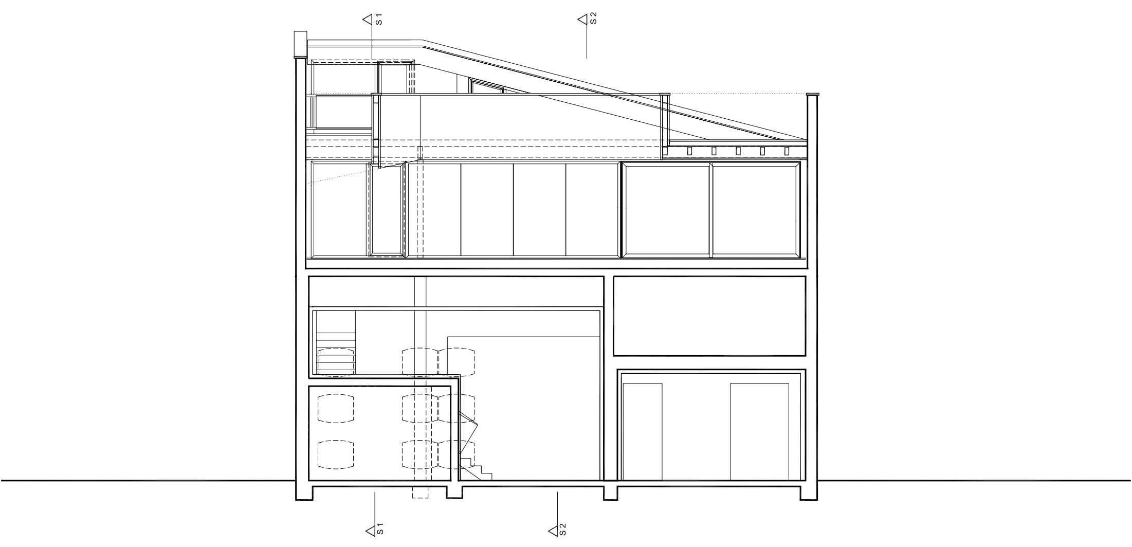
Schnitt 3
