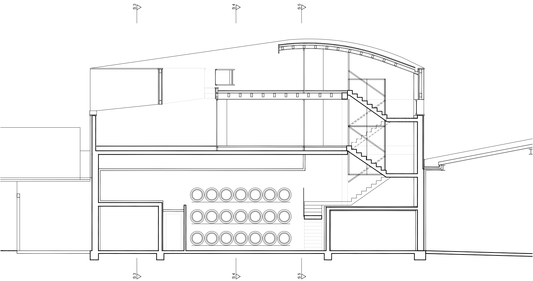
Schnitt 1
