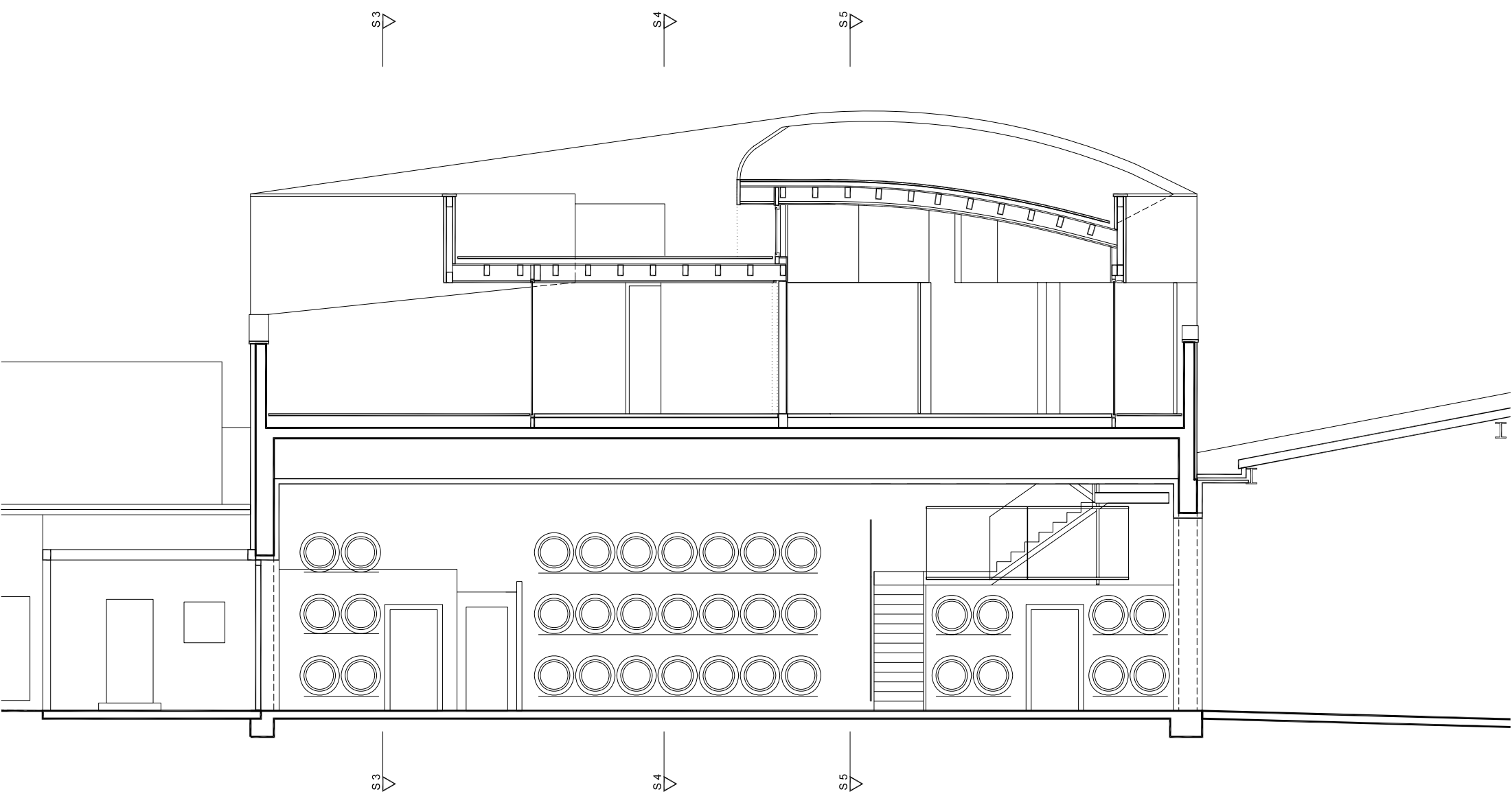
Schnitt 2
