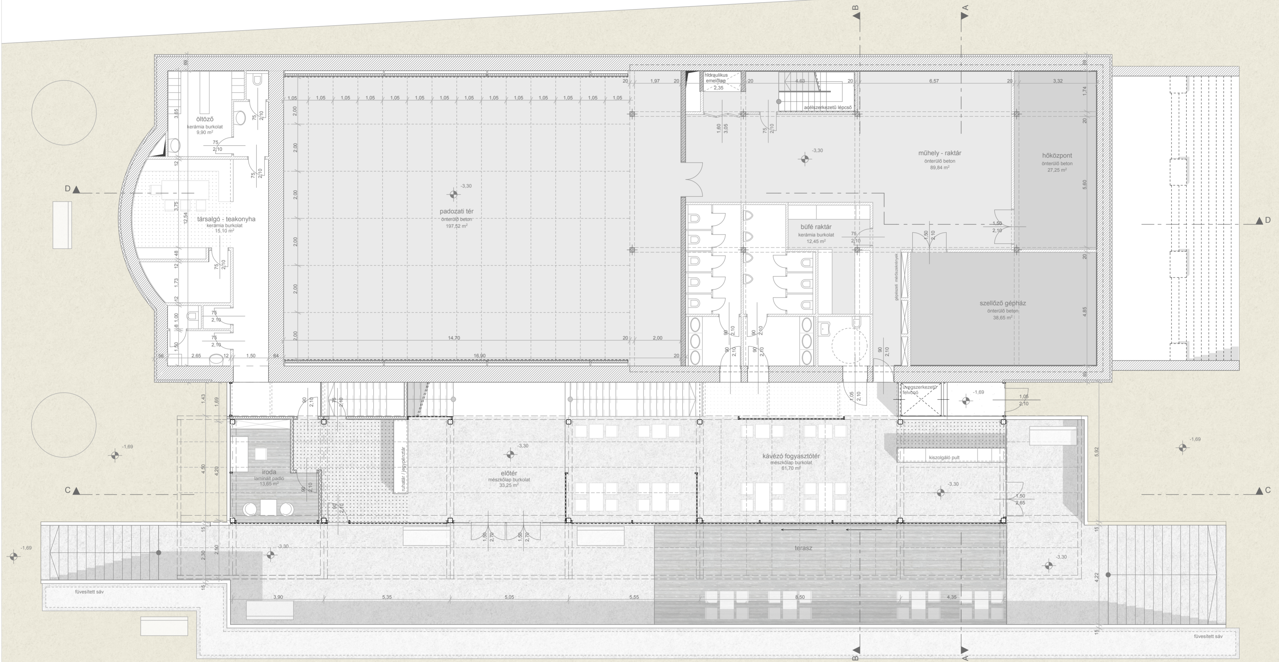
alsó szint alaprajza m = 1 : 100
