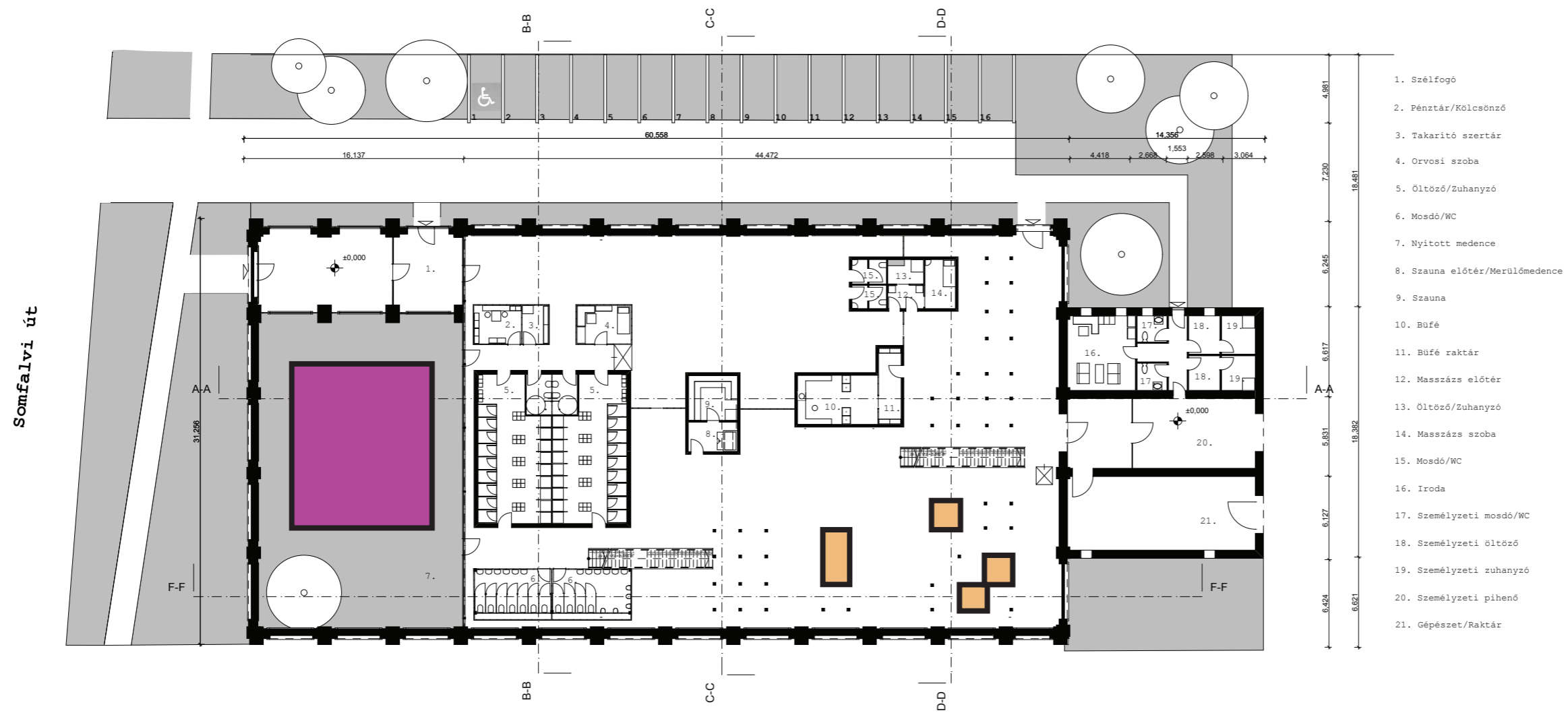
Földszinti Alaprajz ↗
