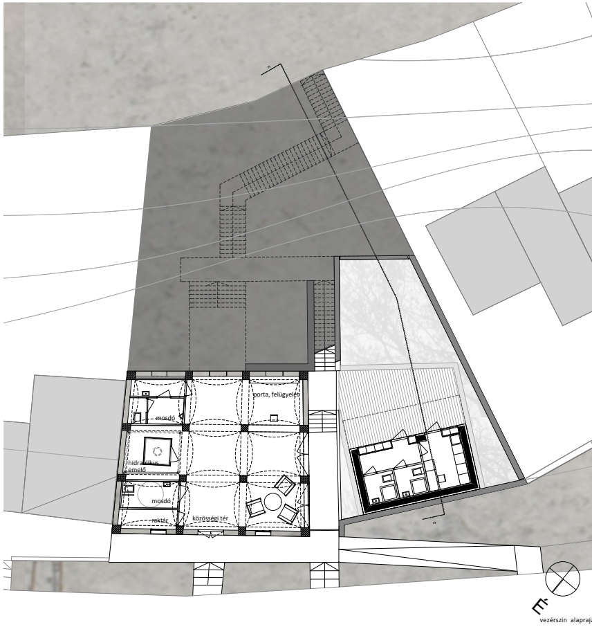
vezérszín alaprajz
