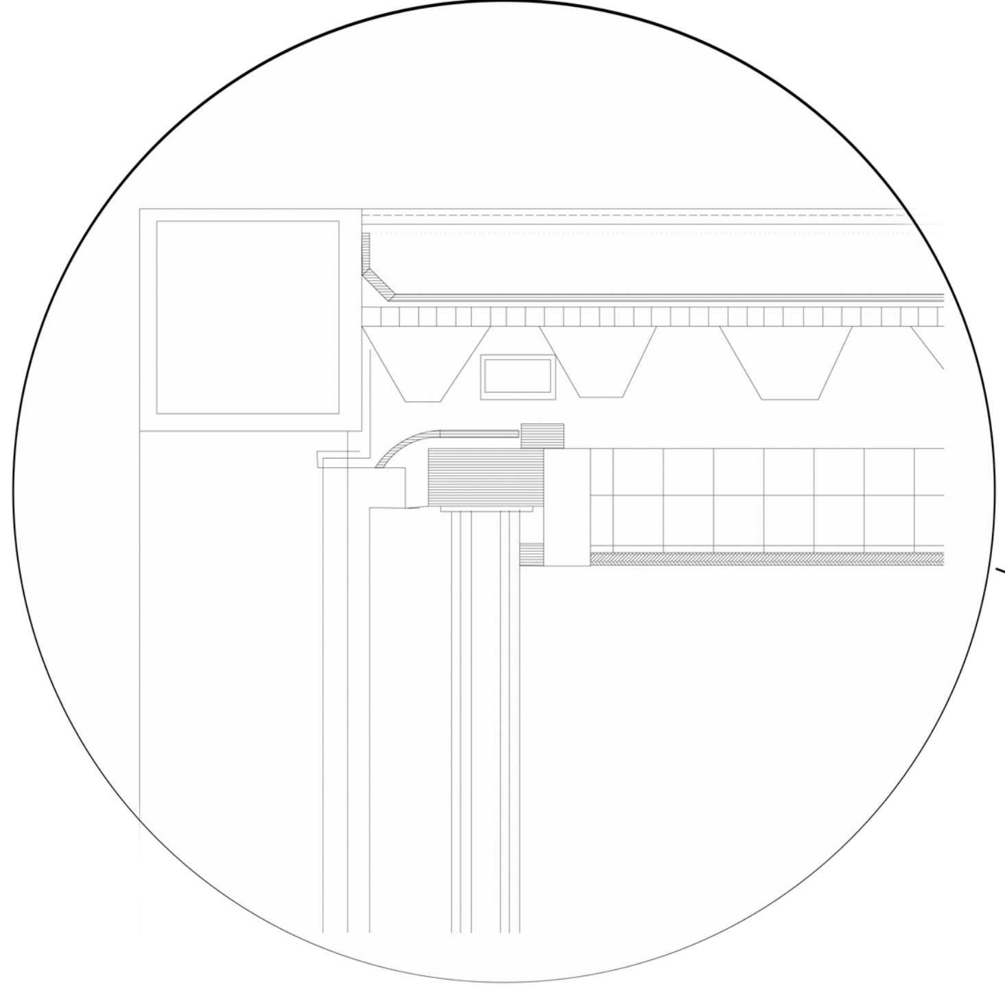
MŰHELY ÜVEGFAL CSOMÓPONT
