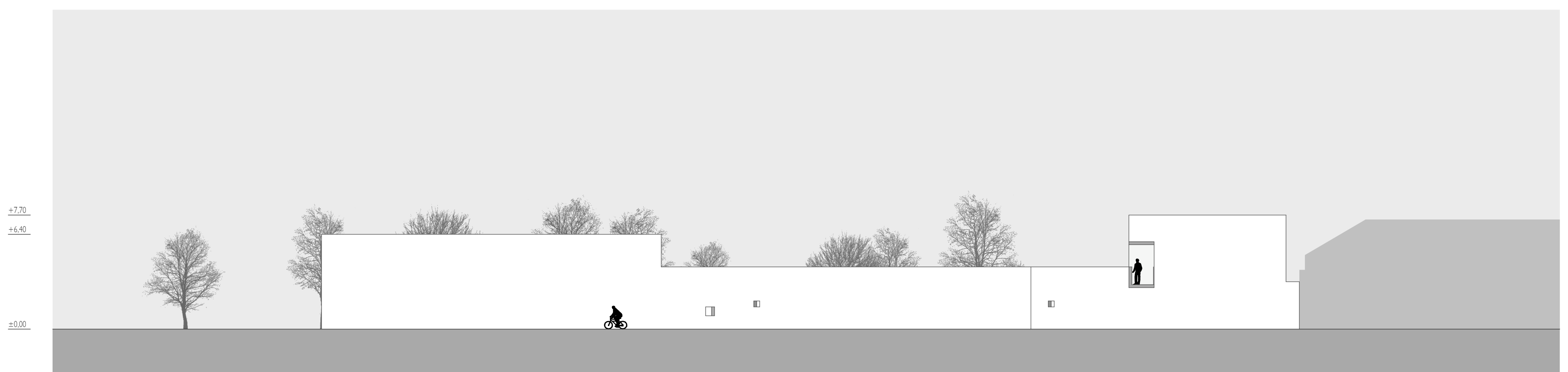
keleti homlokzat
