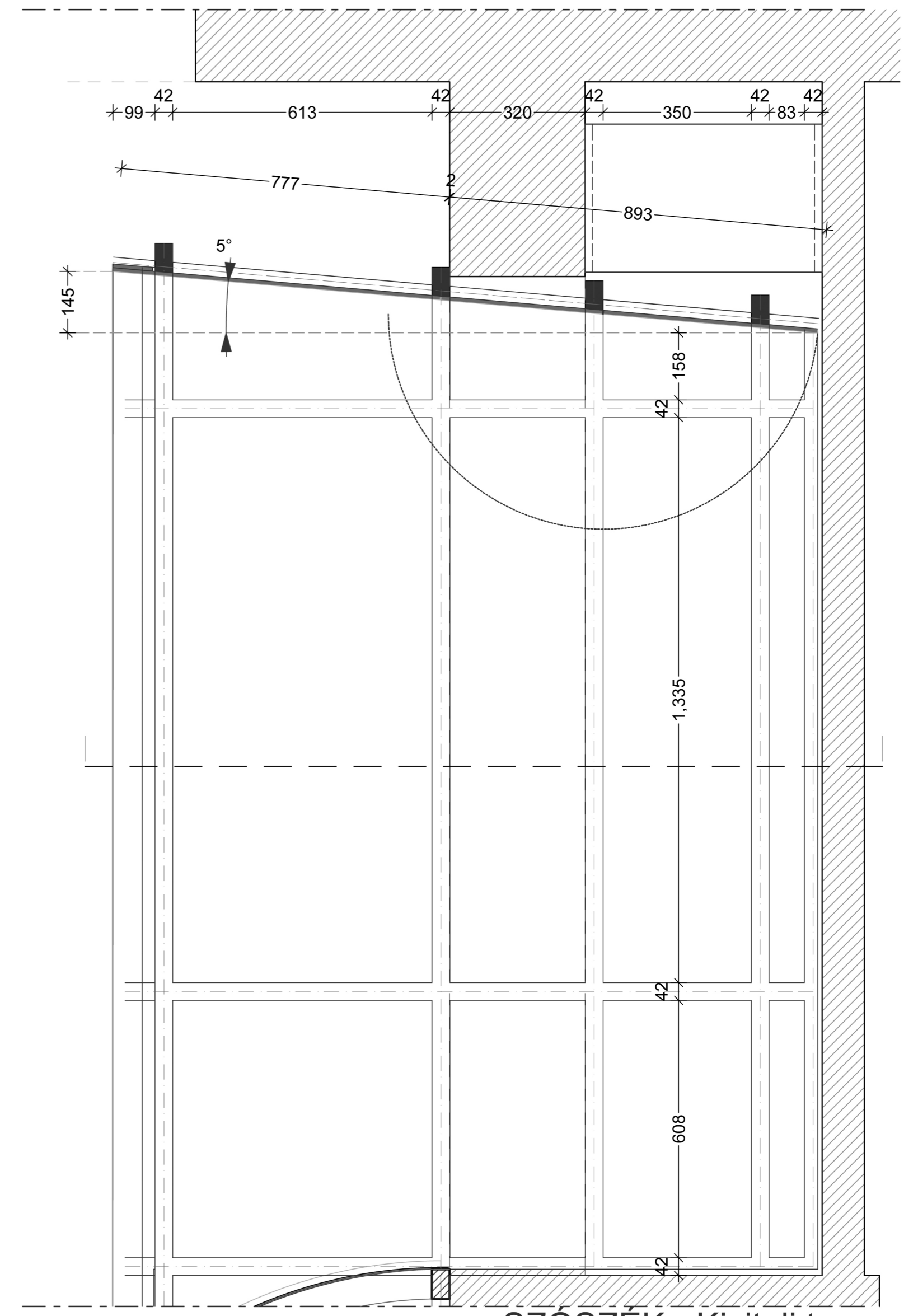
SZOSZÉK - Kiviteli terv A-A Metszet, homlokzati nézet, alaprajzi részlet M=1:10 Csepel - Királyerdő - Református gyülekezeti ház ifj Szakál Ferenc Csorba Réka 20110217
