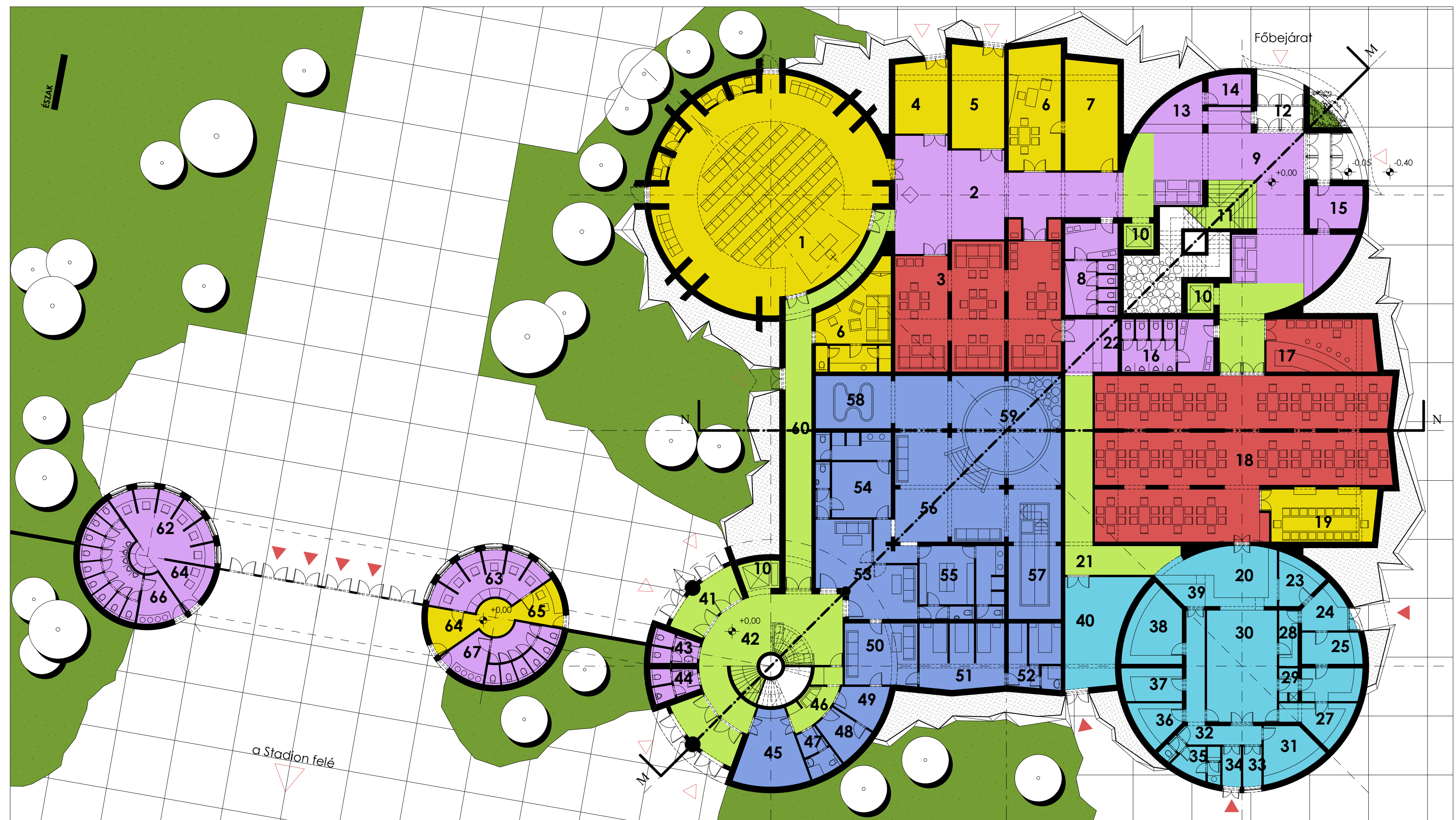
FÖLDSZINTI ALAPRAJZ lépték 1:200
