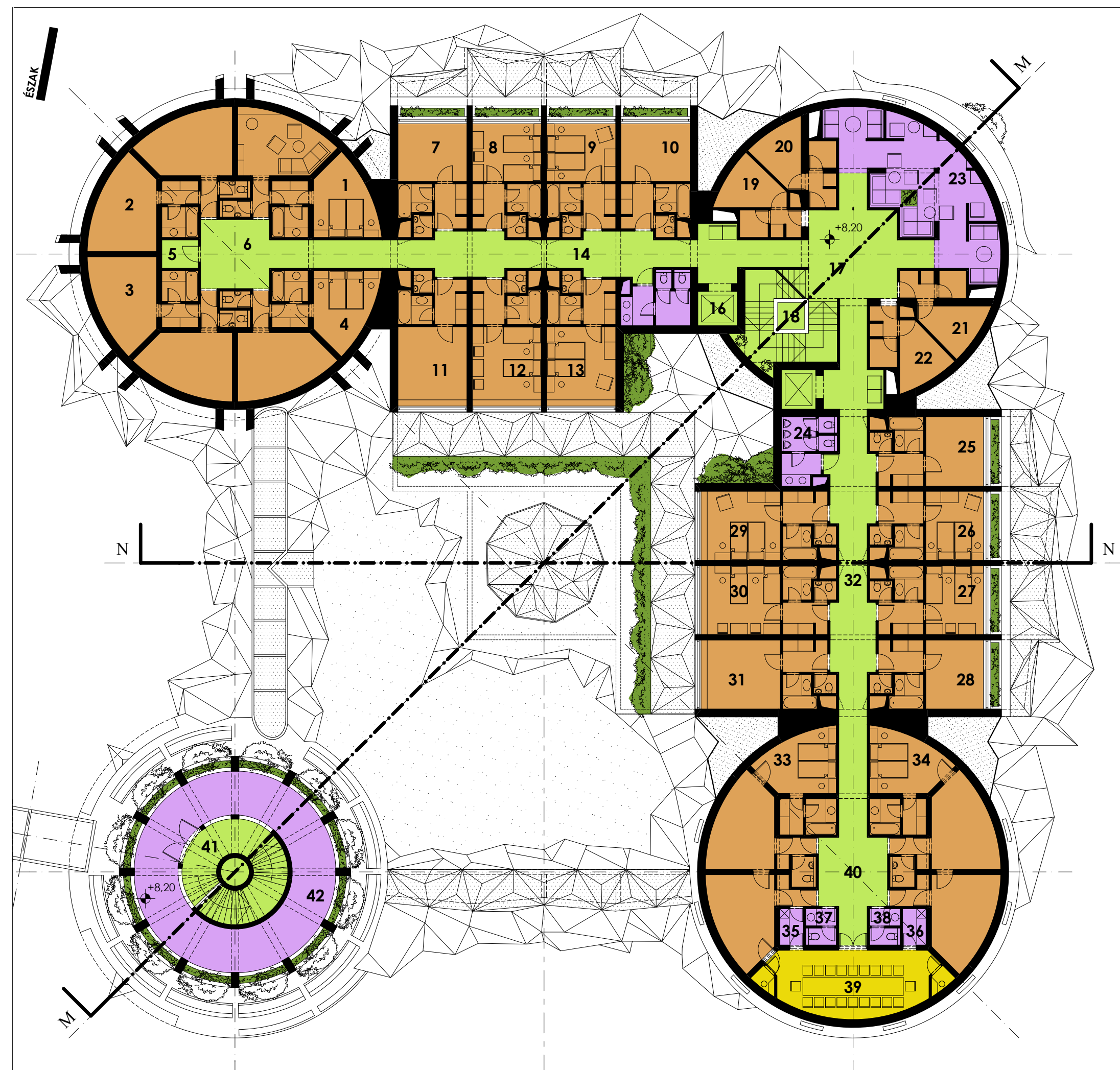
MÁSODIK EMELETI ALAPRAJZ lépték 1:200
