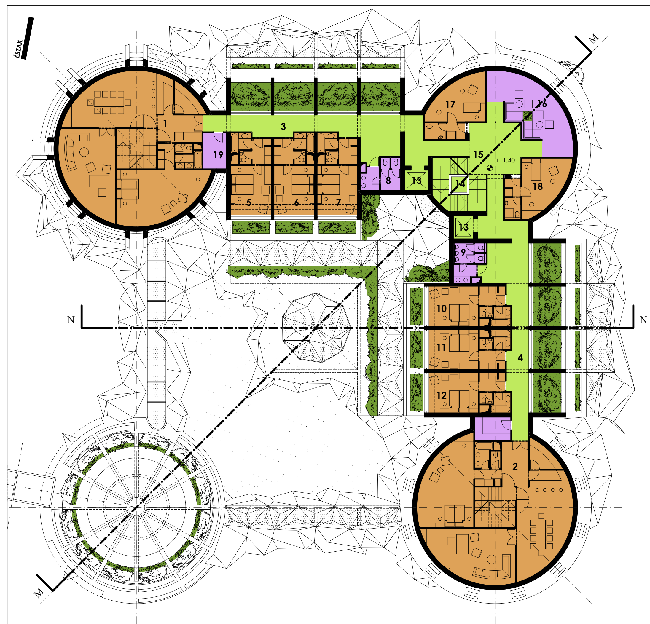
HARMADIK EMELETI ALAPRAJZ lépték 1:200
