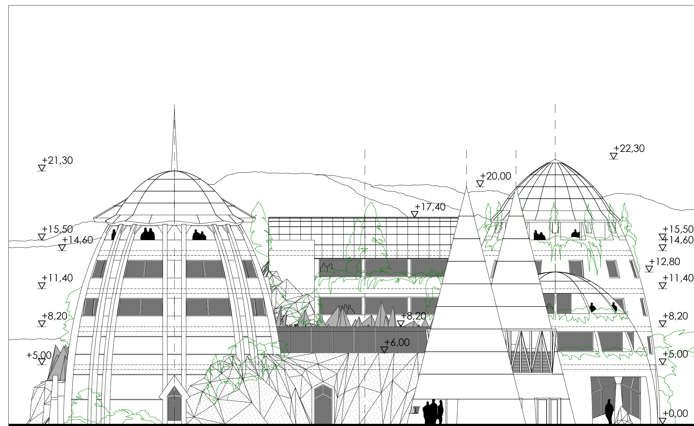
NYUGATI HOMLOKZAT lépték 1:200
