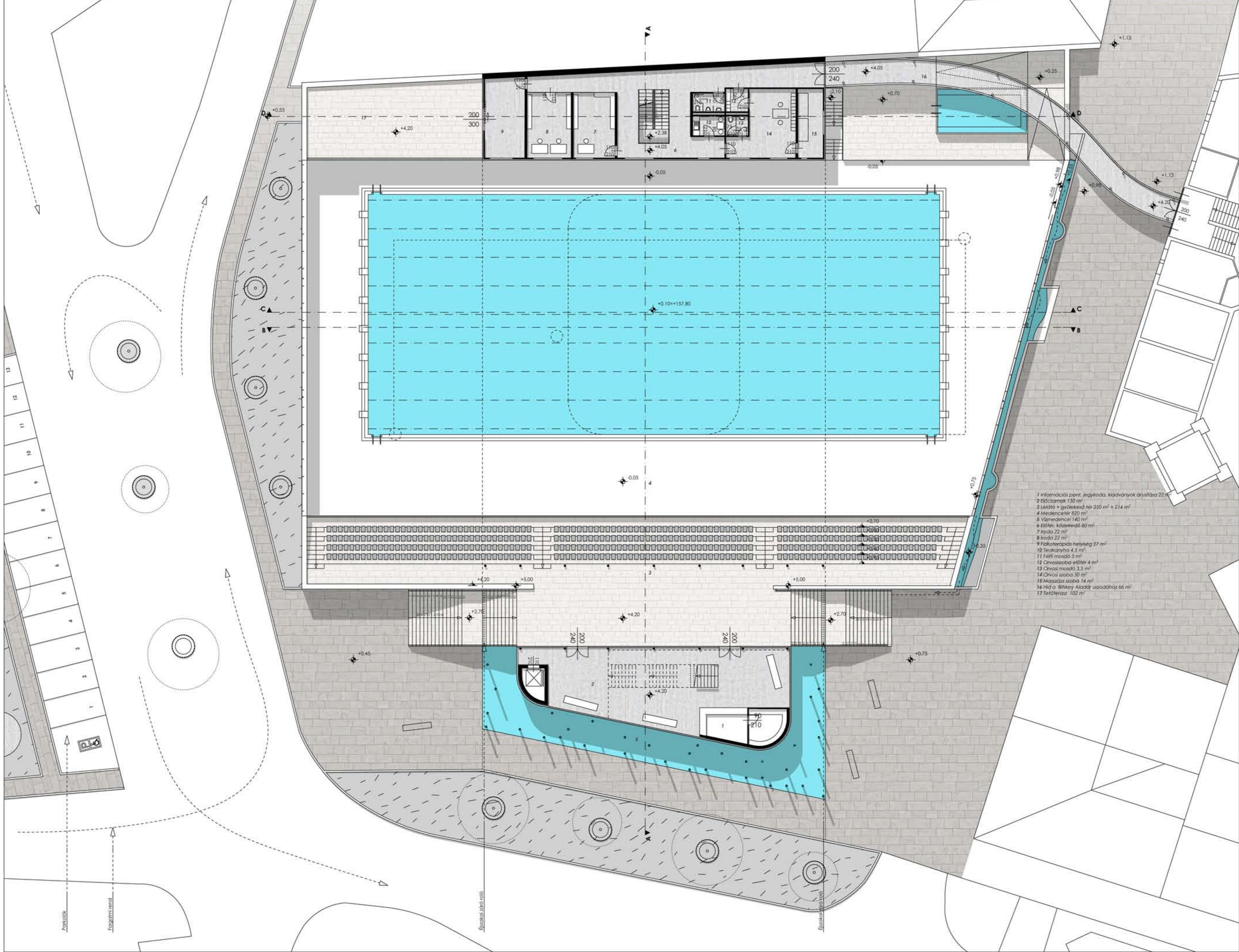
1. emeleti szint alaprajza M=1:200
