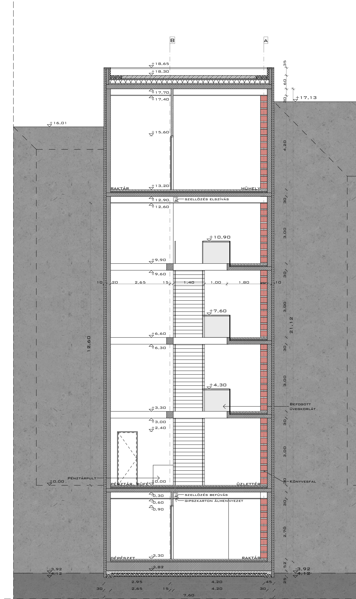
C-C METSZET
