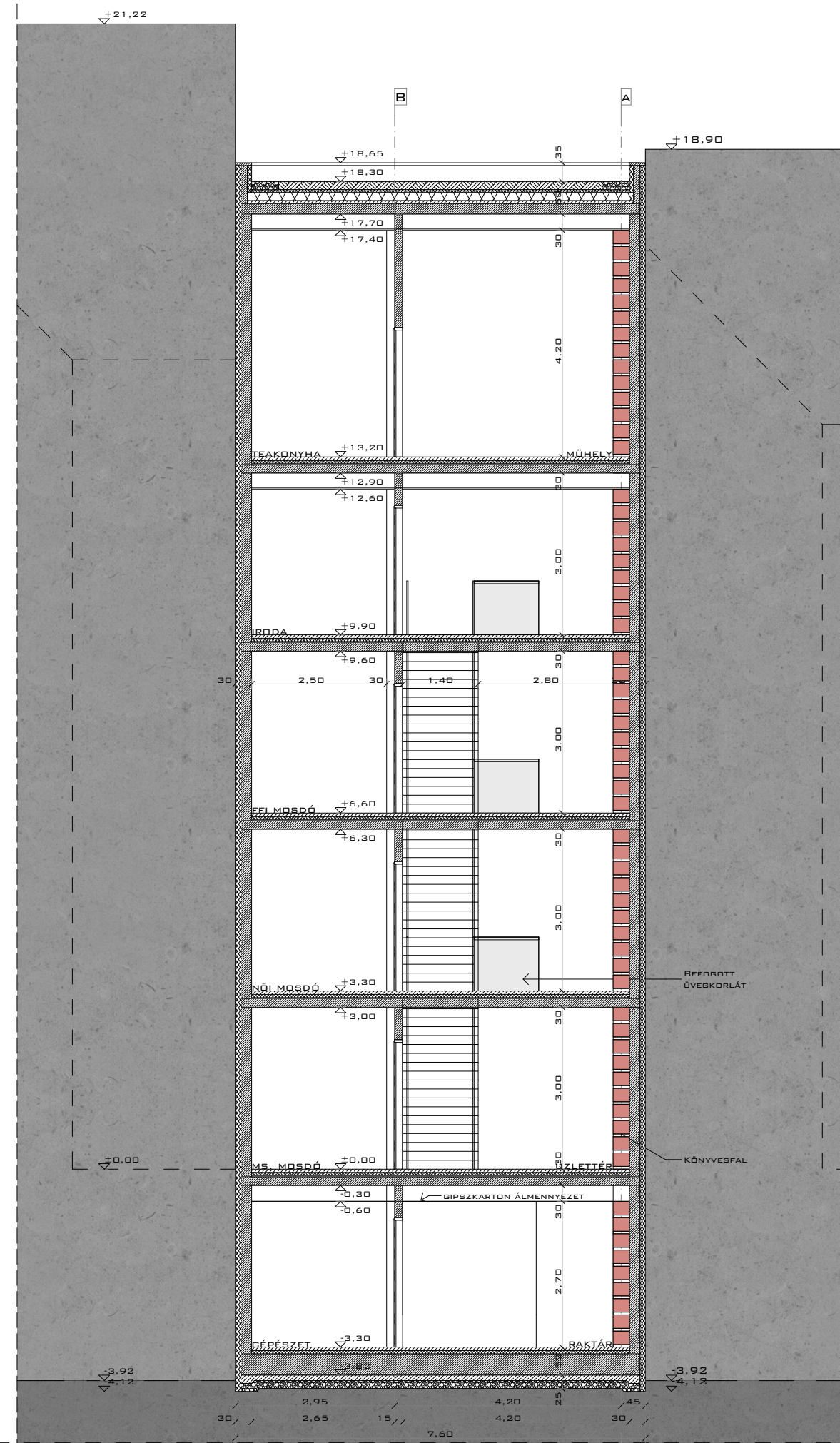
B-B METSZET
