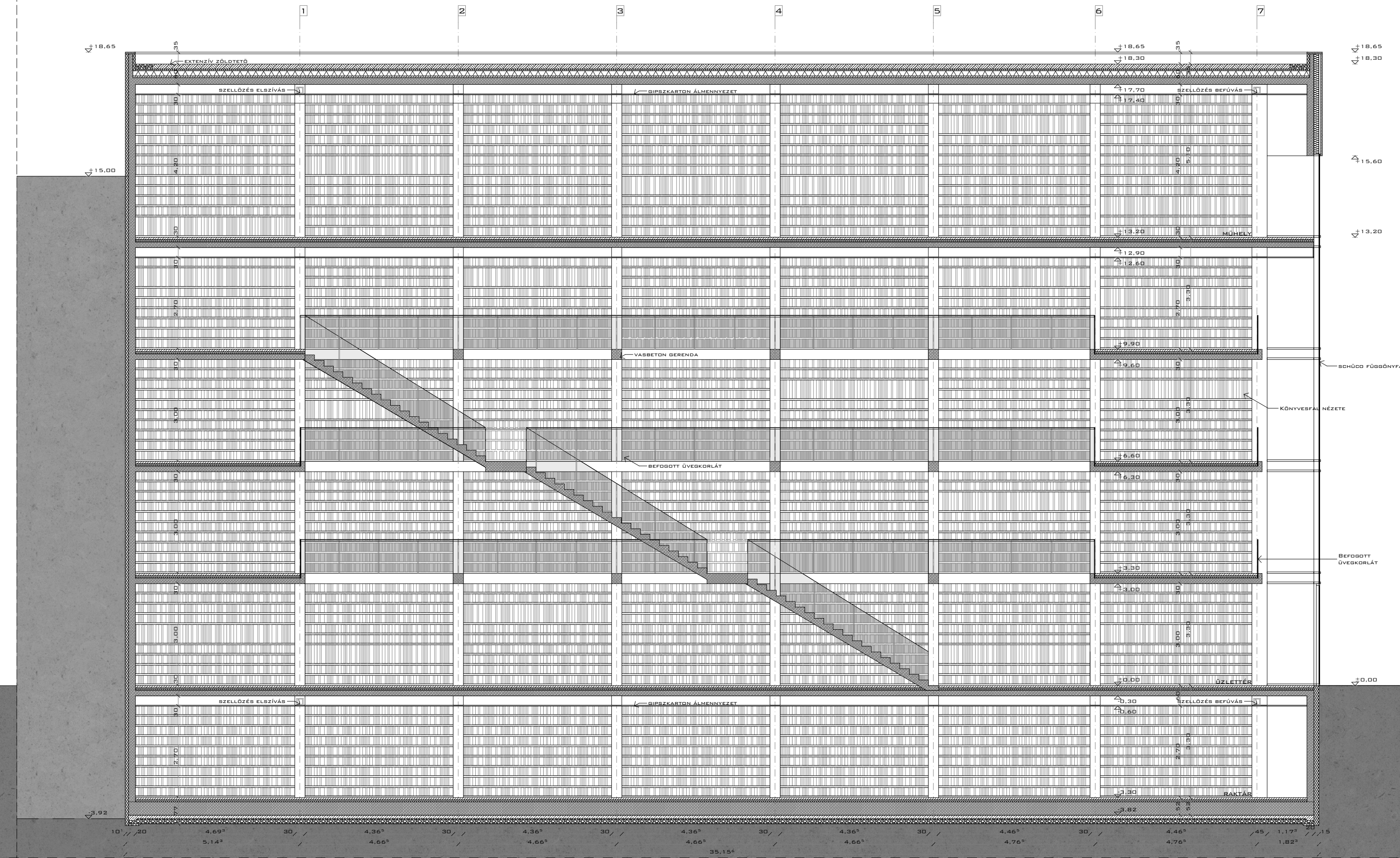
G-G METSZET
