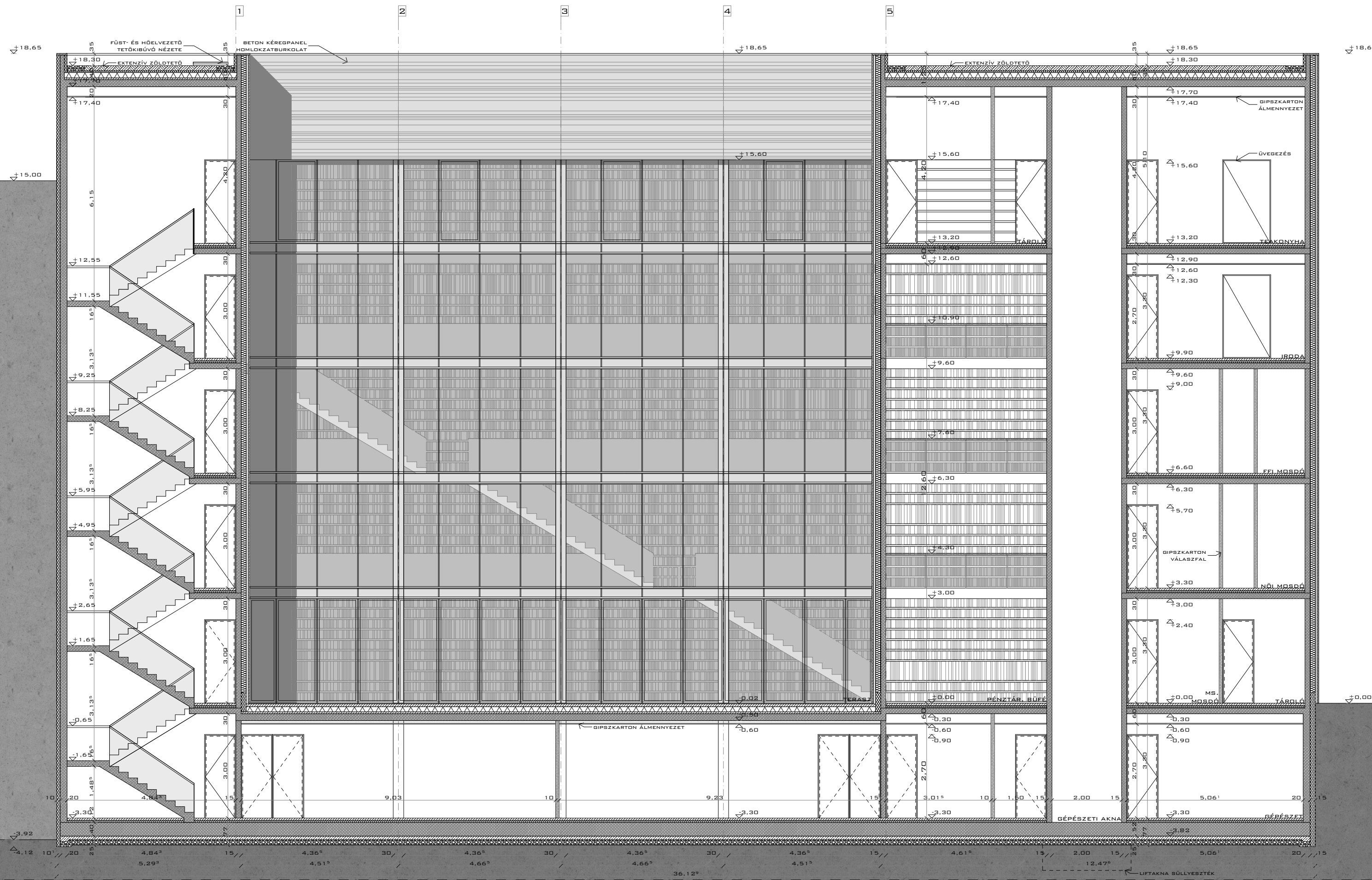
F-F METSZET
