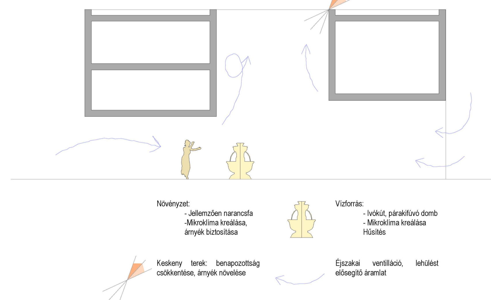
Axonometrikus metszet, a földszinti földem felső síkja felett 1 m-rel felvéve
