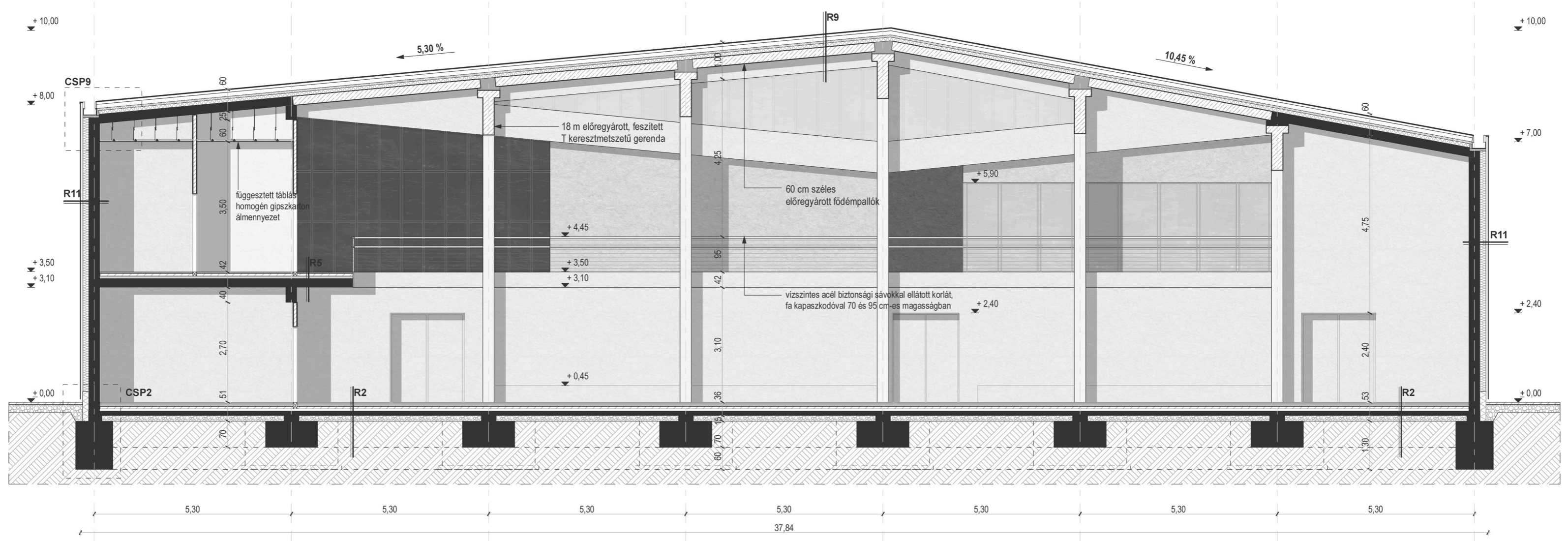
B-B metszet
