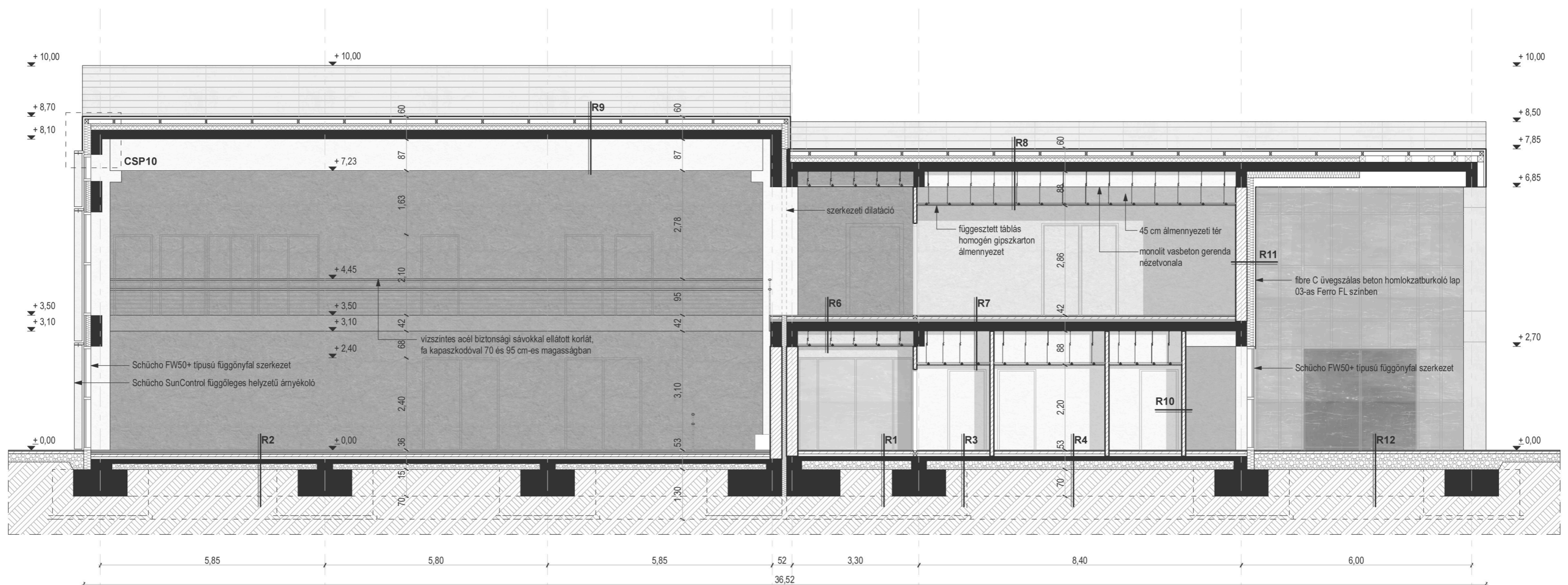
C-C metszet
