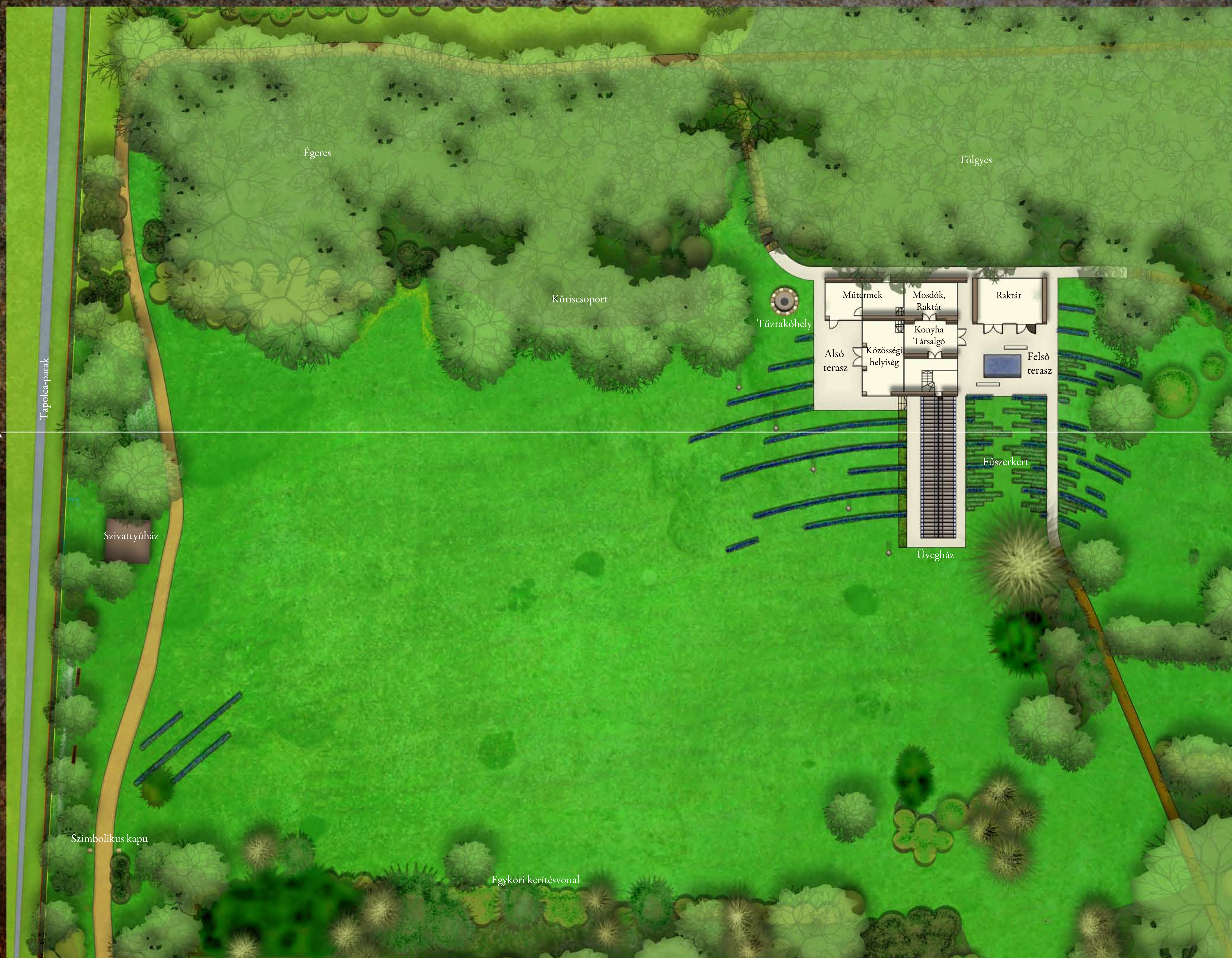
A NAGYRÉT SZABADTÉRÉPÍTÉSZETI TERVE M=1:250
