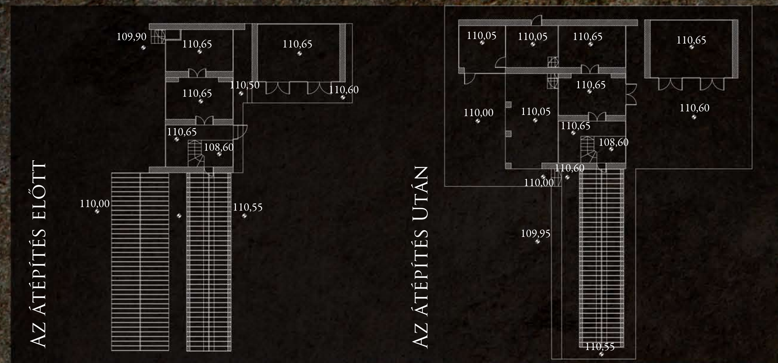
AZ ÜVEGHÁZ ÉS A KAPCSOLÓDÓ ÉPÜLETEK ÁTÉPÍTÉSI TERVE M=1:200
