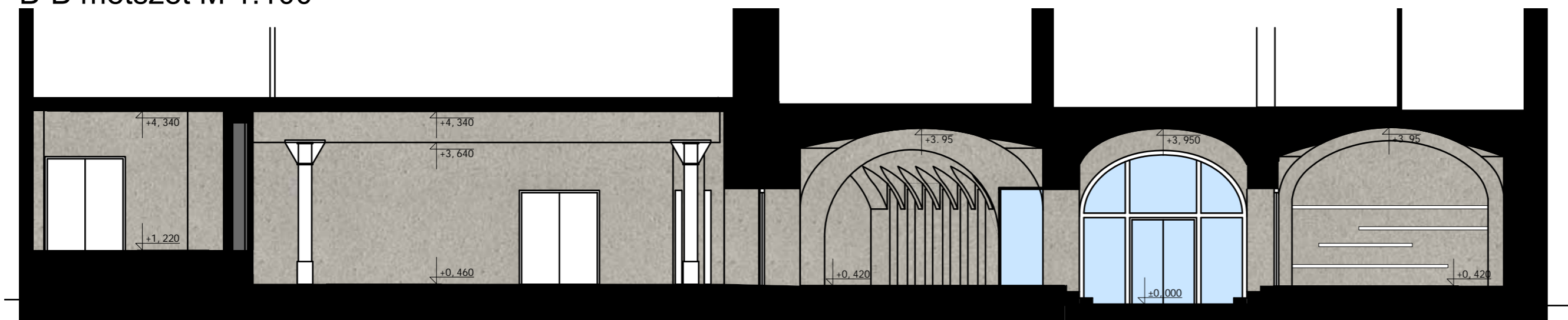
B-B metszet M 1:100
