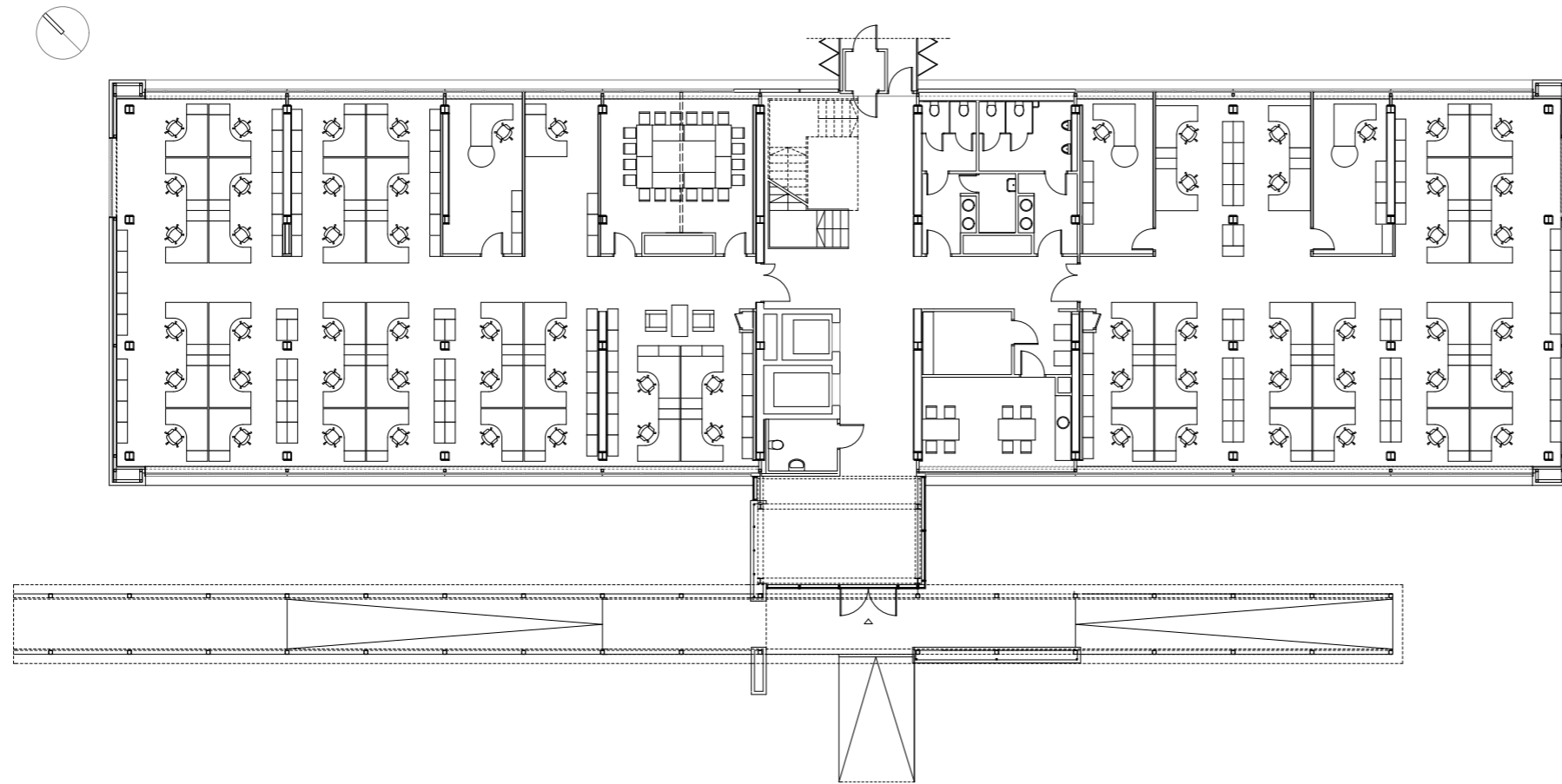
BUDAPEST AIRPORT 72. A-C ÉPÜLET FÖLDSZINTI ALAPRAJZ
