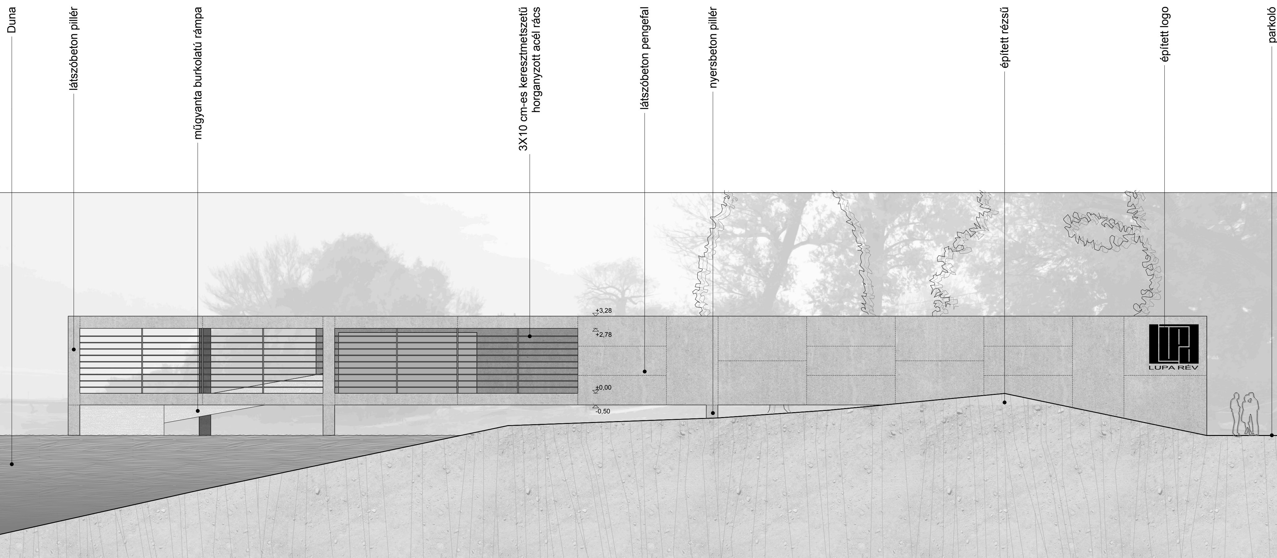
északi homlokzat
