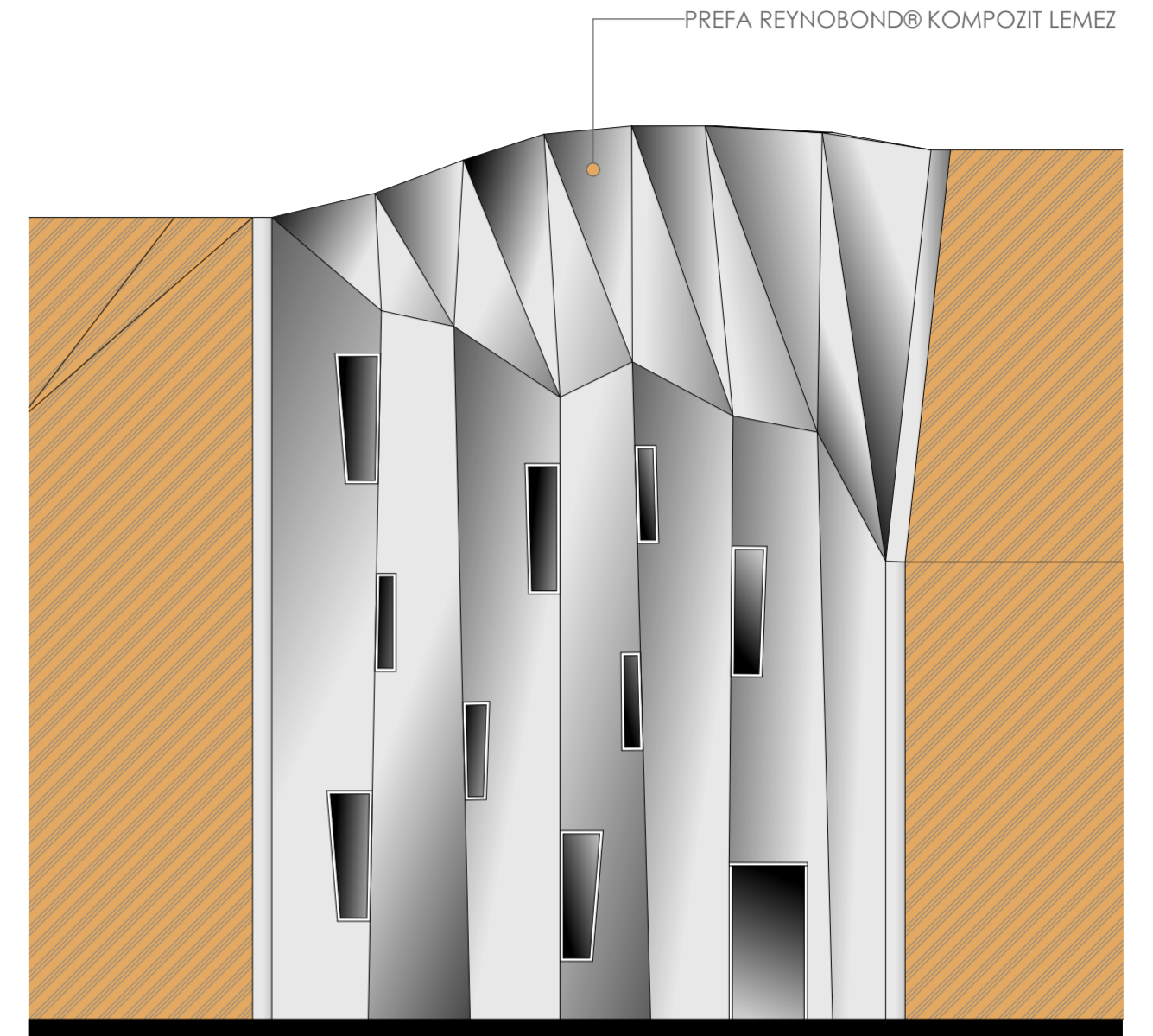
DÉL-KELETI HOMLOKZAT M 1:100
