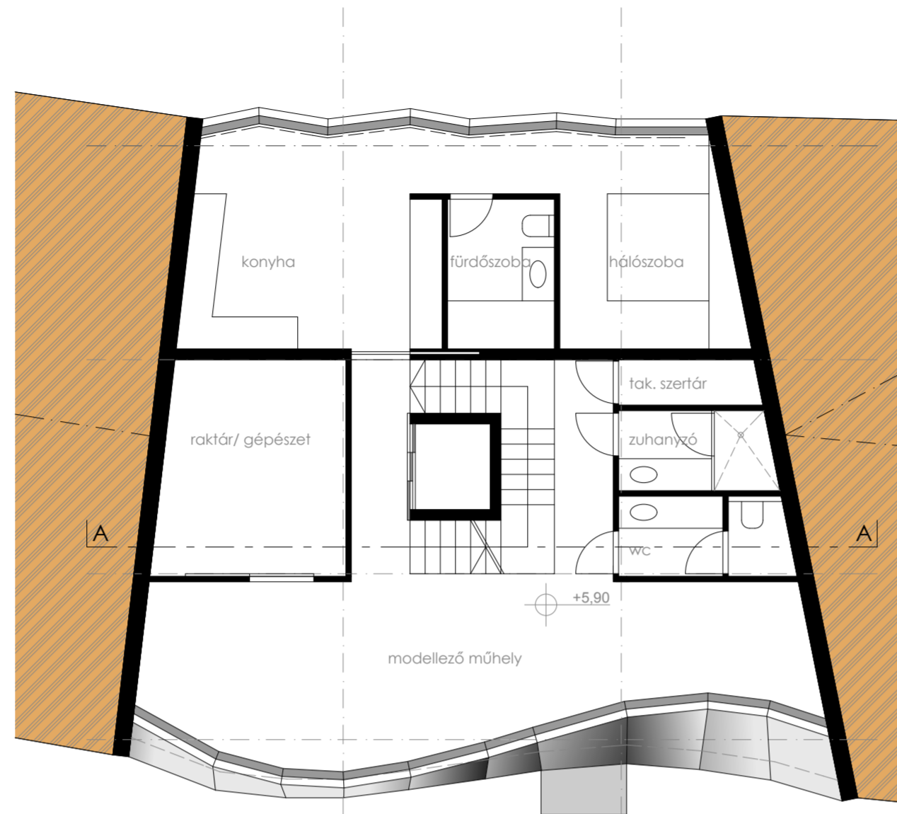
2. EMELETI ALAPRAJZ M 1:100
