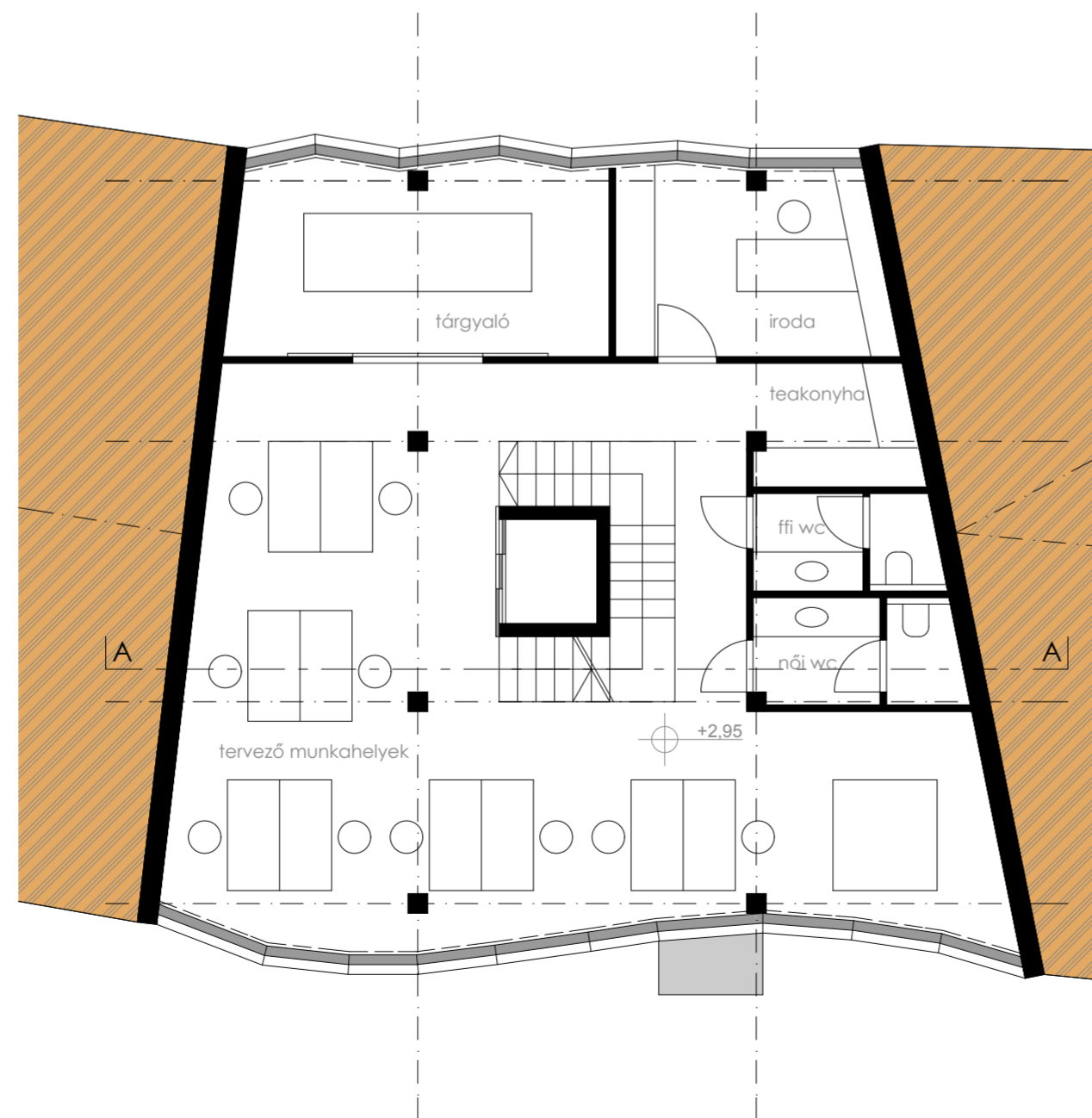
1. EMELETI ALAPRAJZ M 1:100
