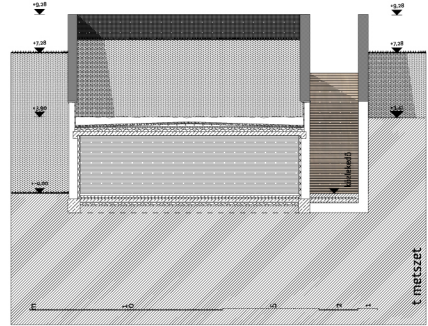
t metszet
