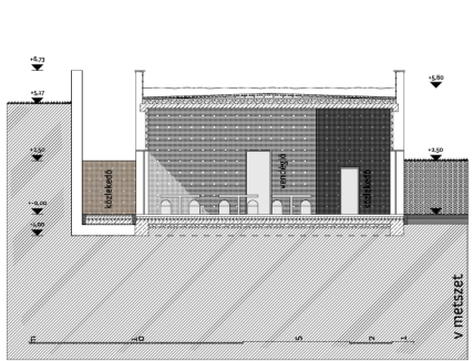
v metszet
