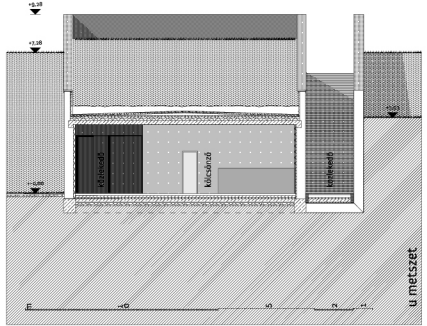
u metszet
