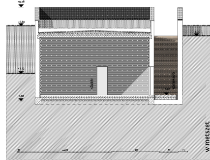
w metszet
