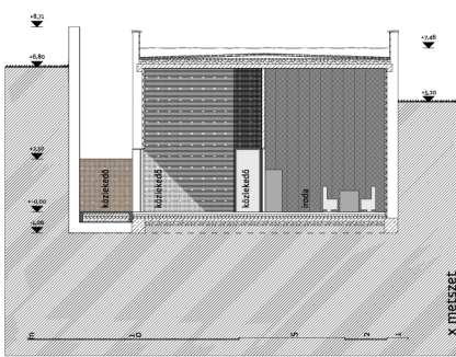
x metszet
