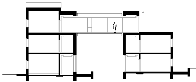
b-b metszet
