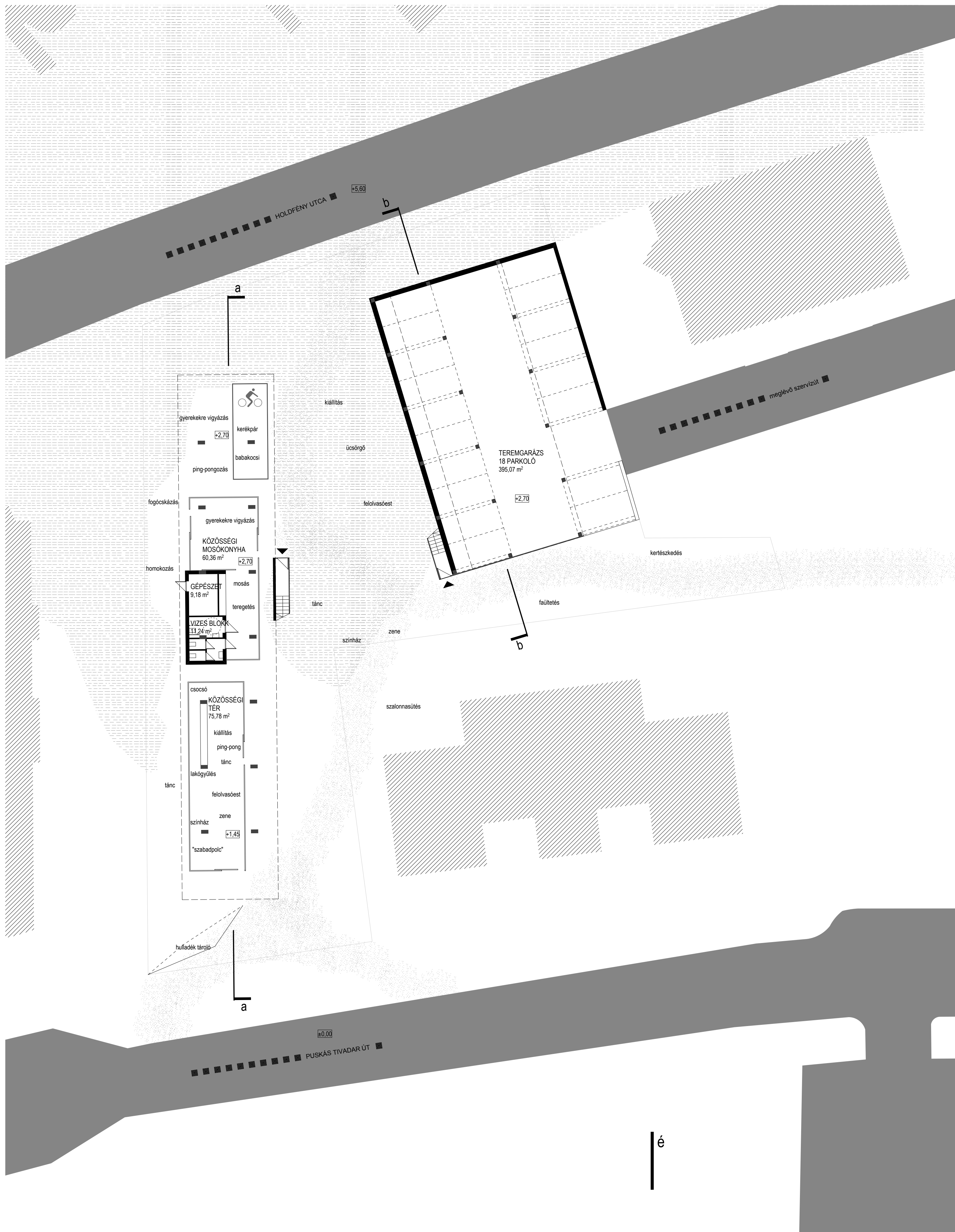
terepszint alaprajz_1:200
