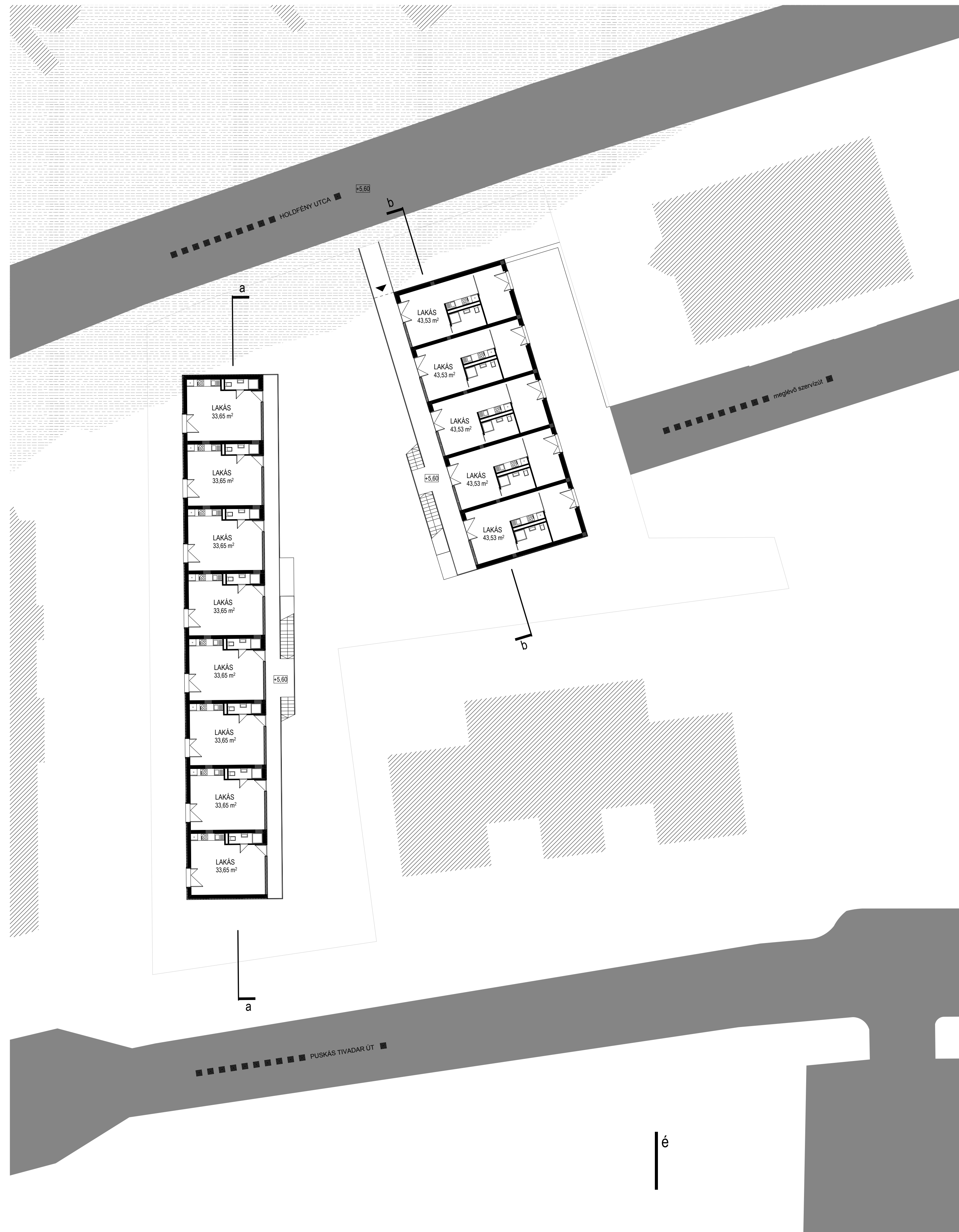
földszint alaprajz_1:200
