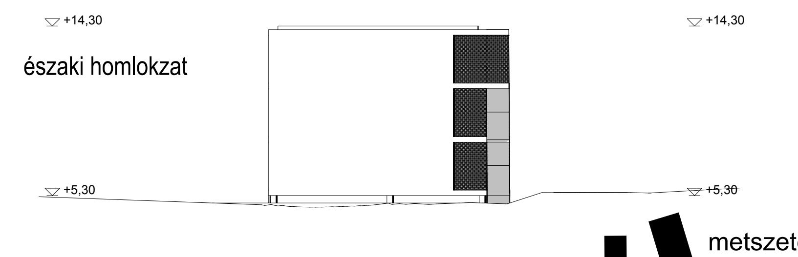
északi homlokzat
