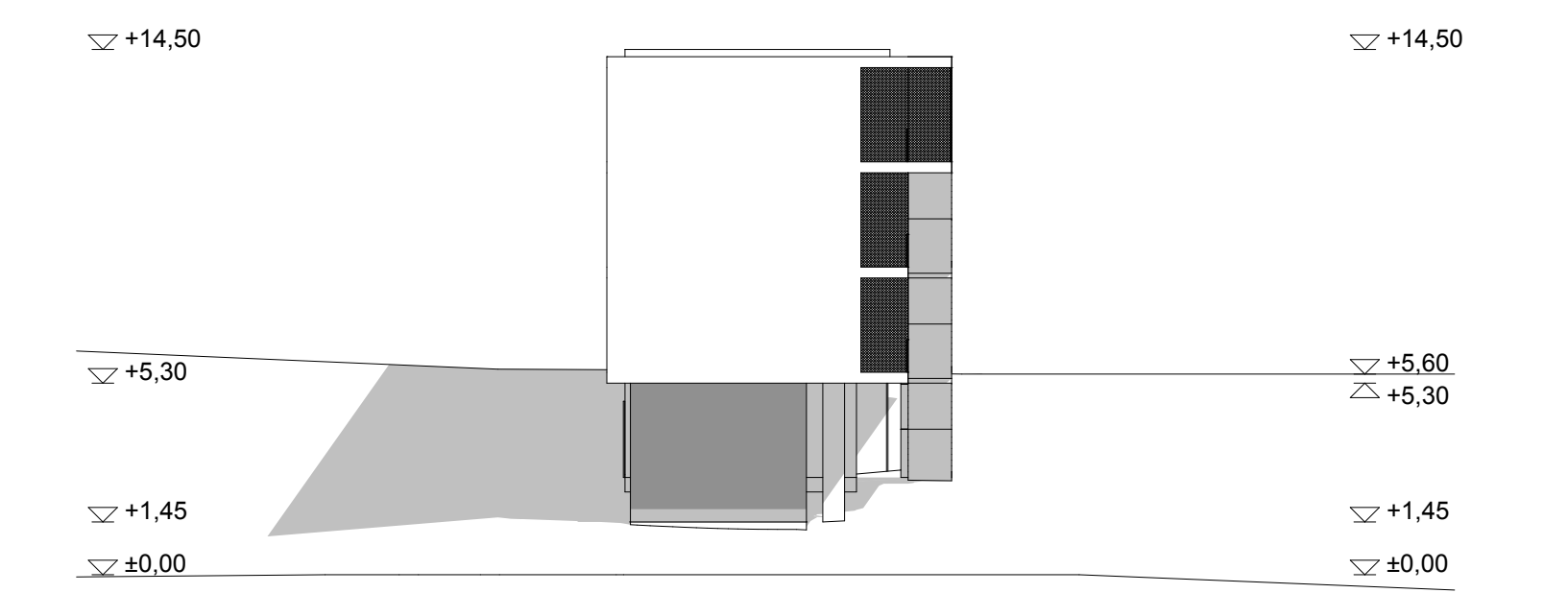
északi homlokzat
