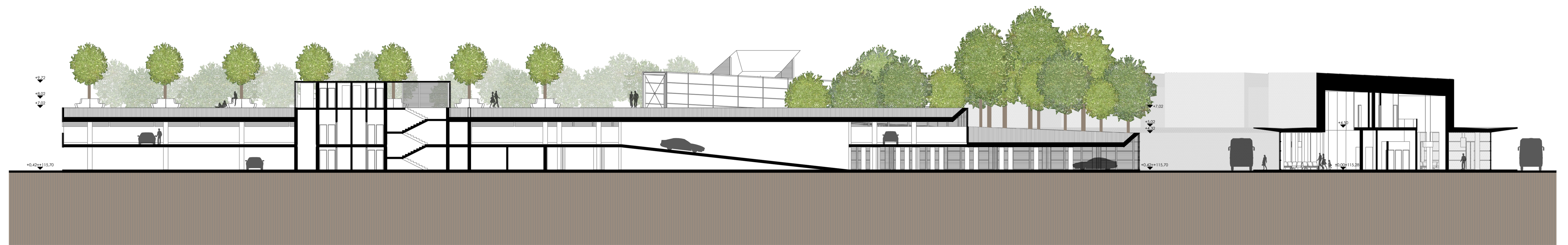
g-g metszet
