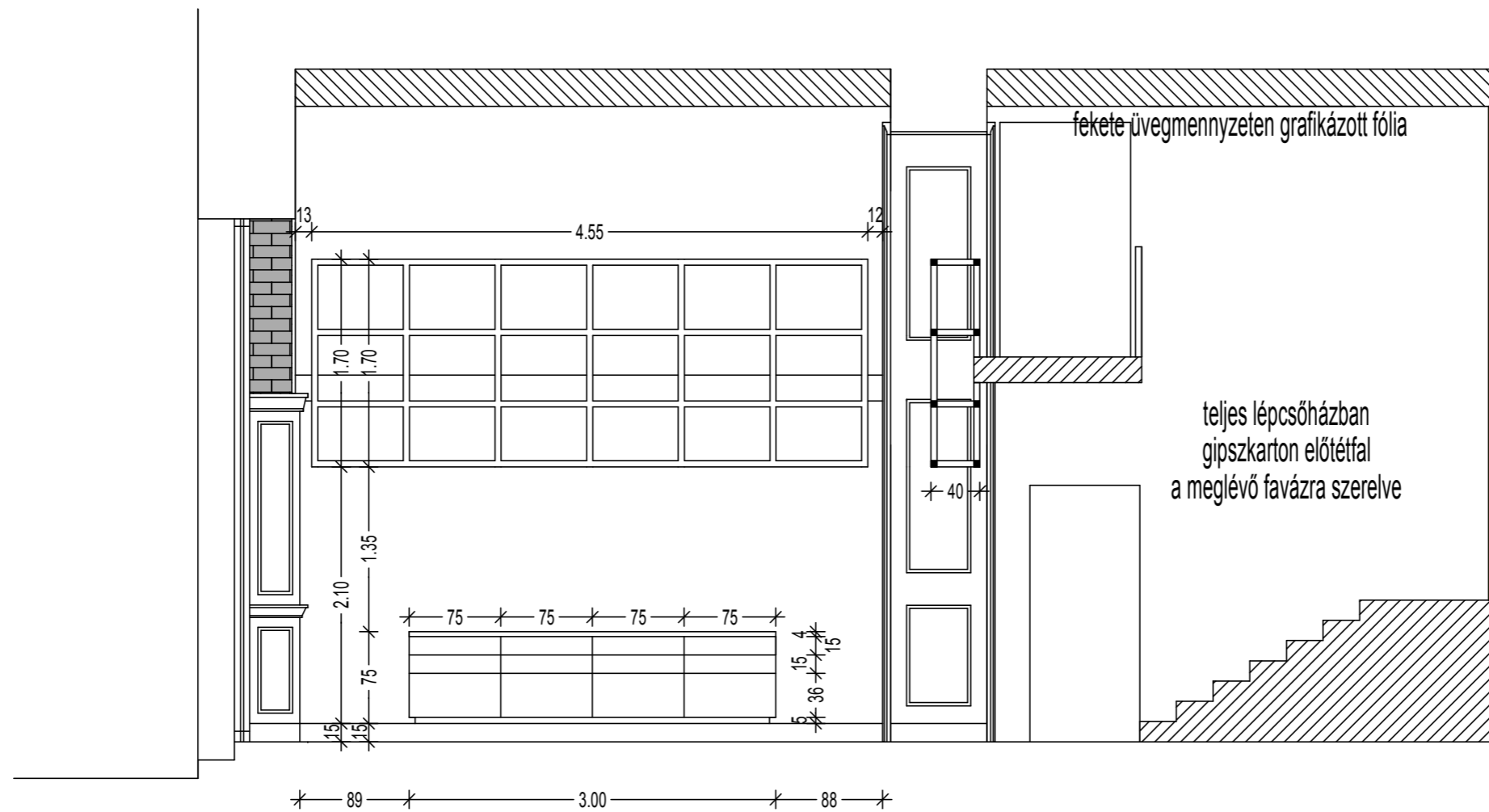
2 - metszet
