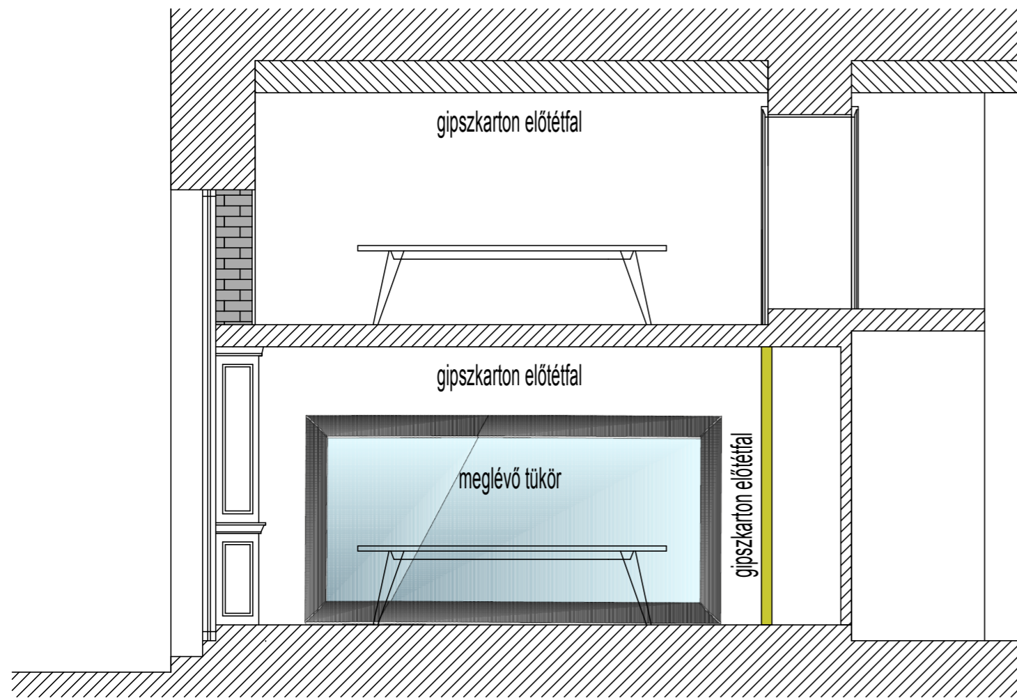
3 - metszet
