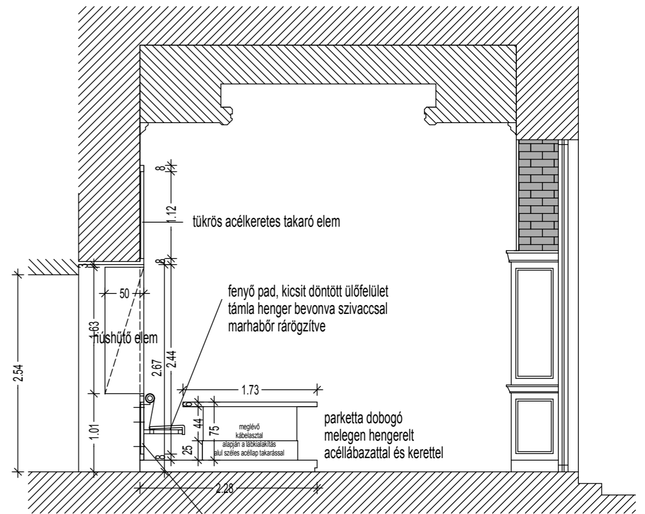
4 - metszet
