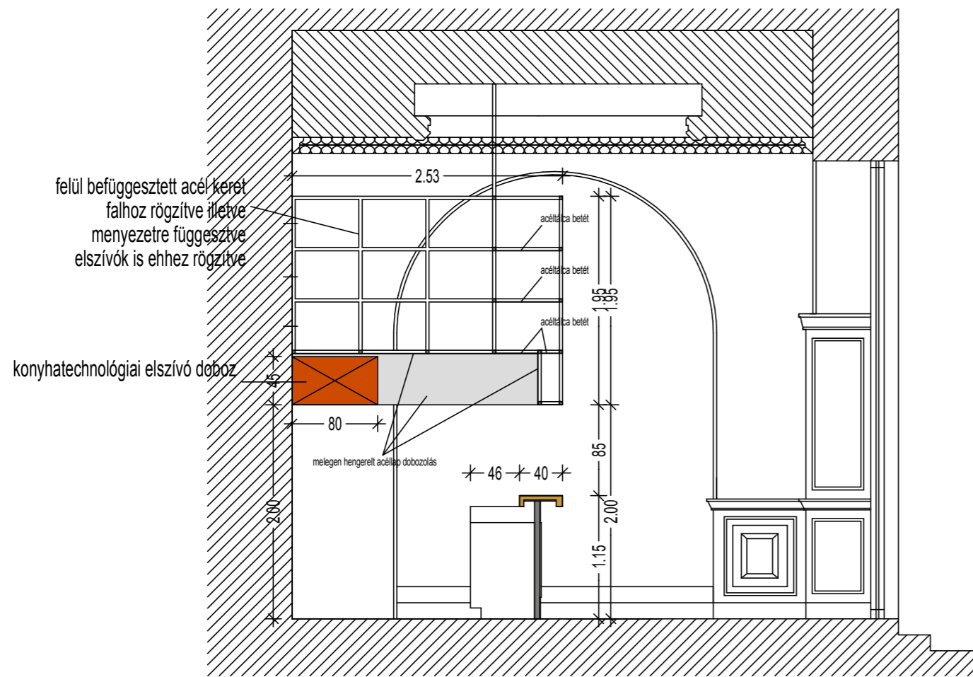
5 - metszet
