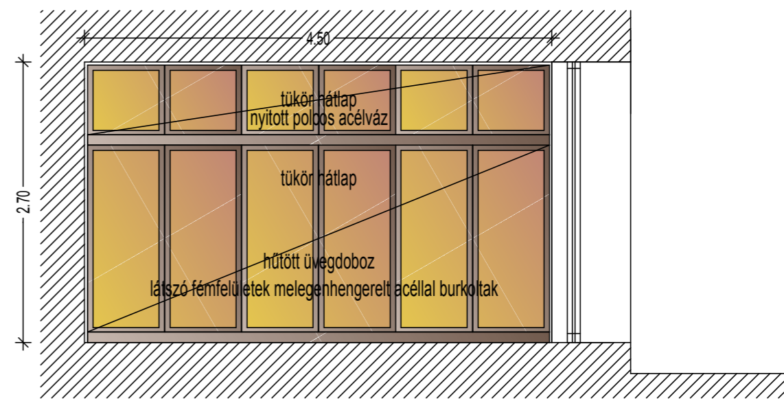
7 - metszet
