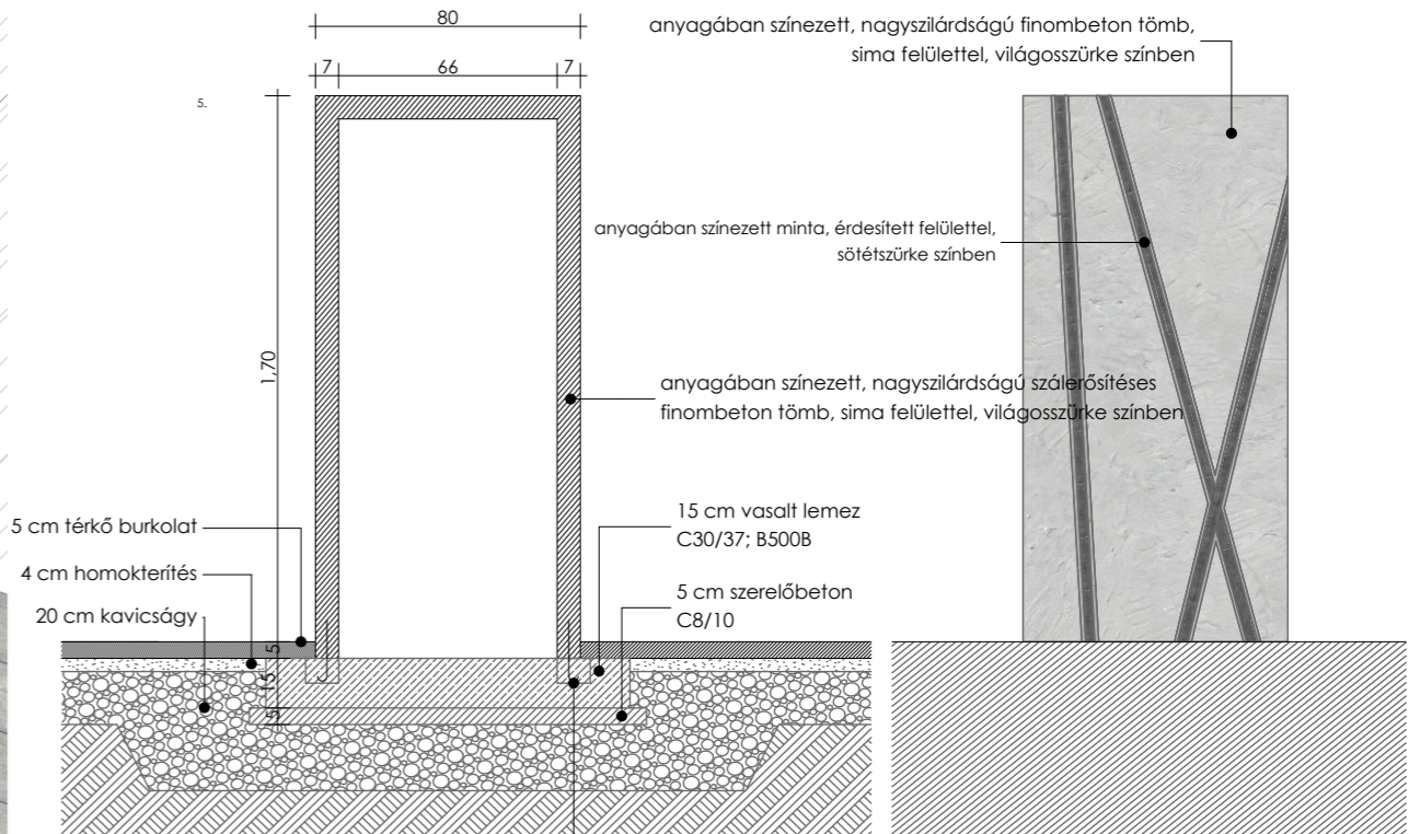
metszet m 1:25
